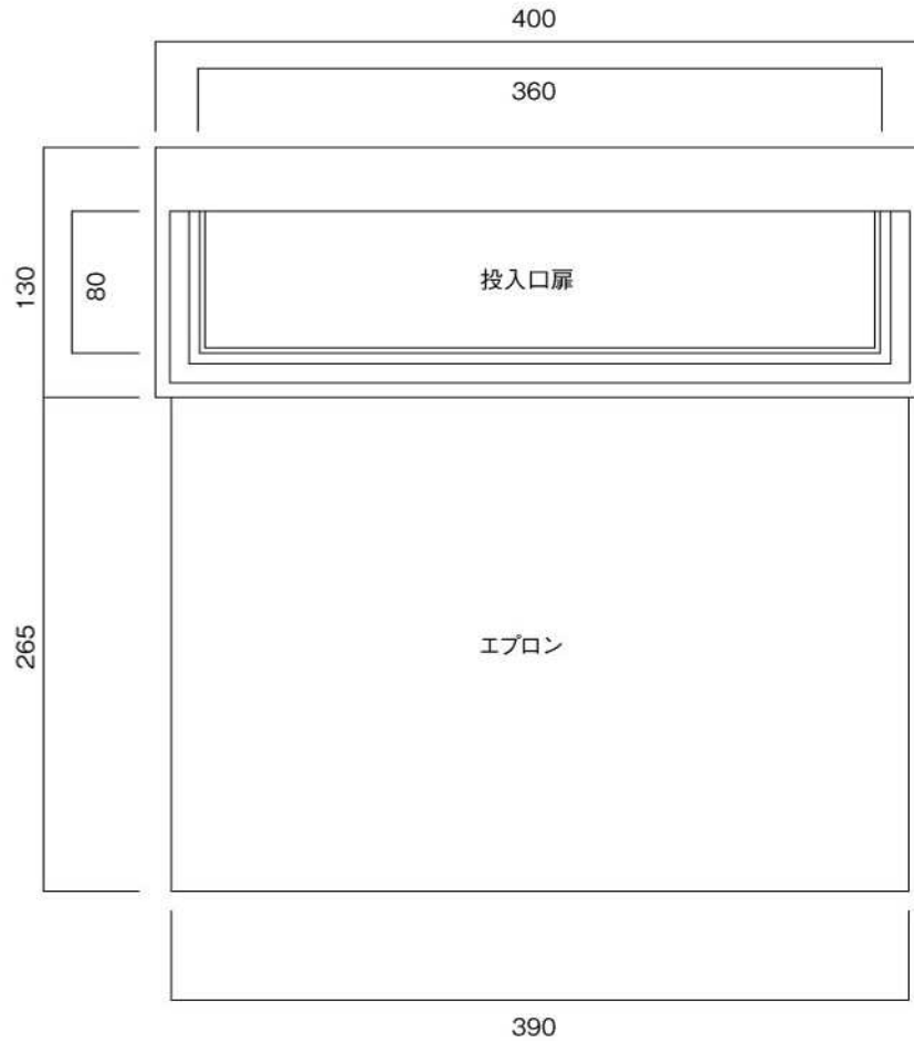
正面図
