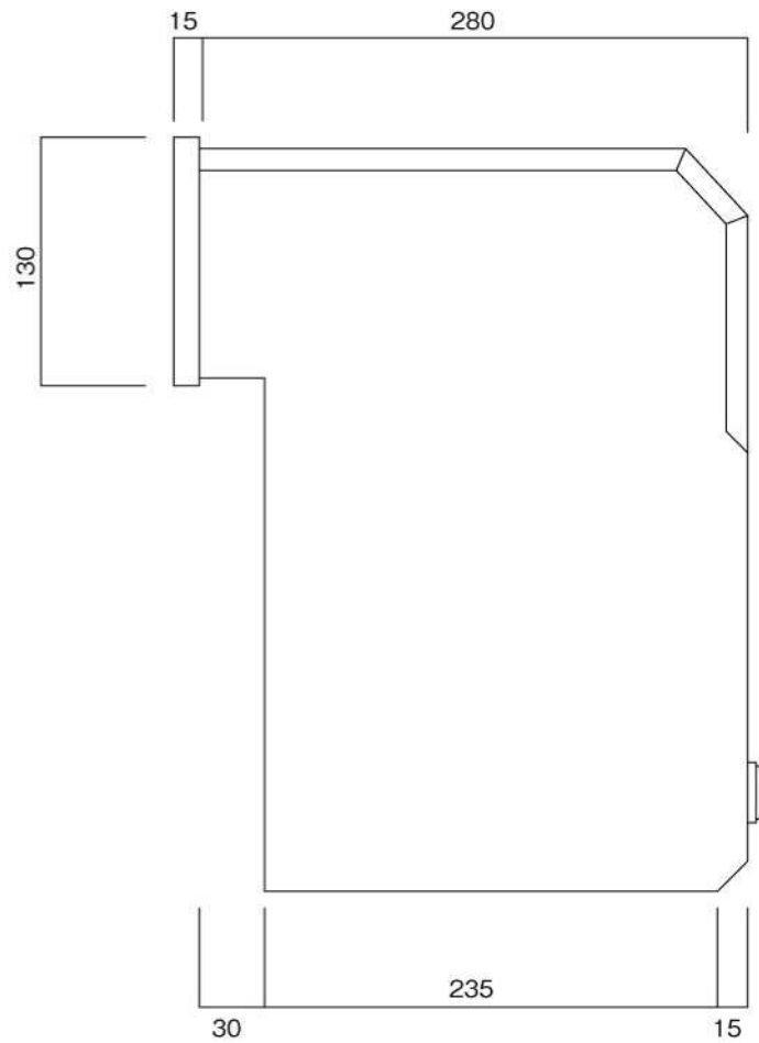
側面図
