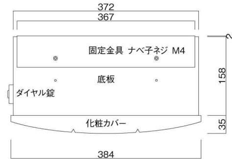
底面図
