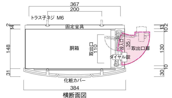
横断面図
