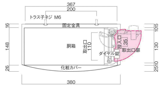
横断面図
