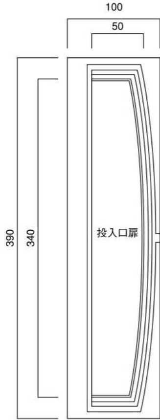
正面図
