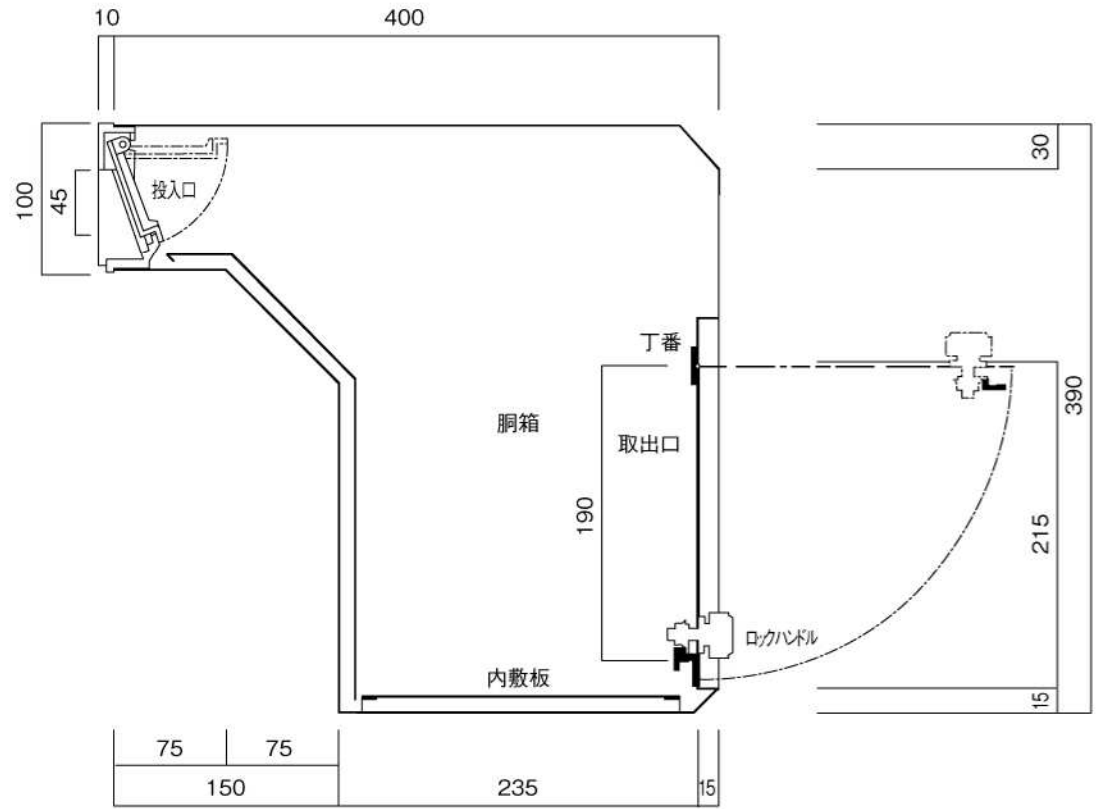
縦断面図
