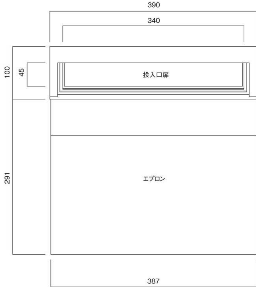
正面図
