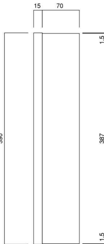
平面図
