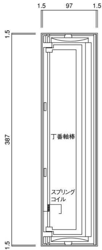
裏面図
