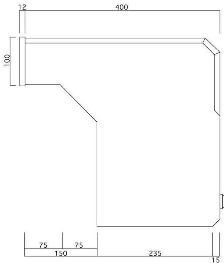
側面図
