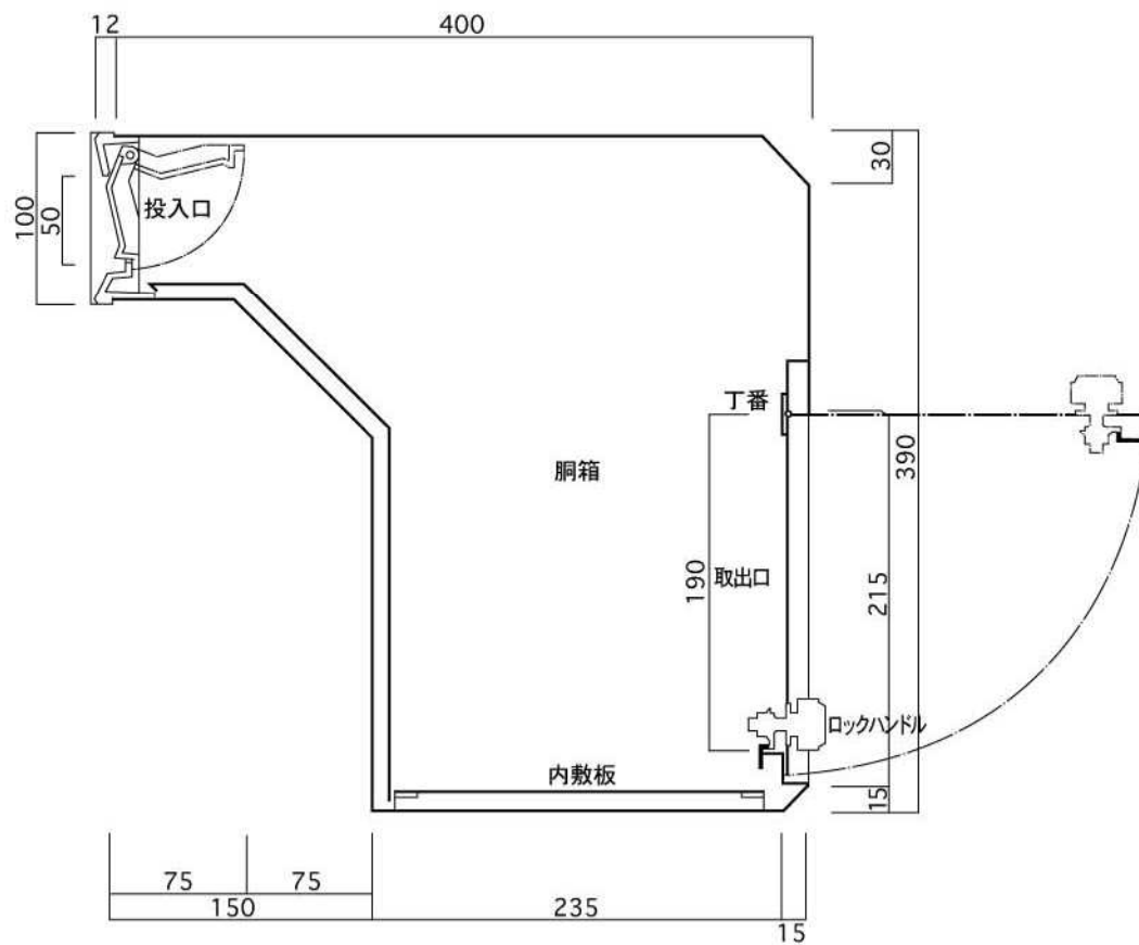
縦断面図
