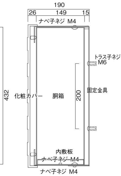
縦断面図
