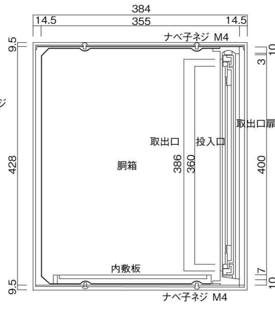
縦断面図
