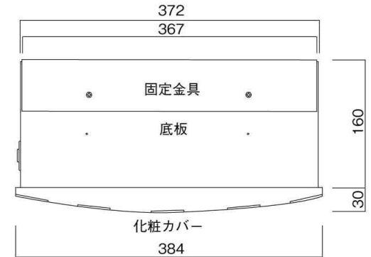
化粧カバー 底面図
