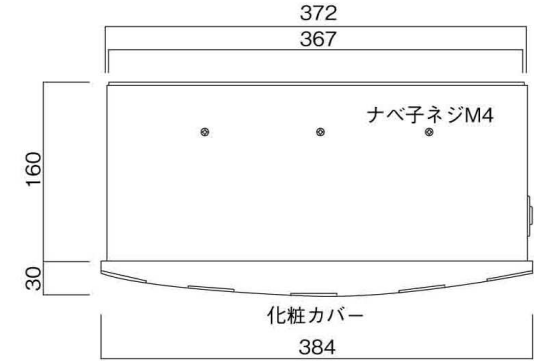
化粧カバー 平面図
