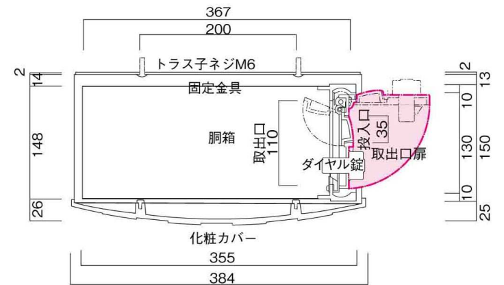
化粧カバー 横断面図
