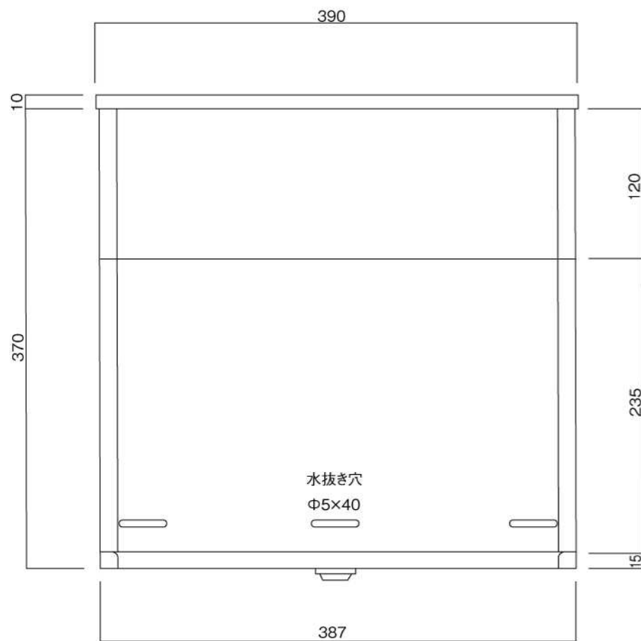
底面図
