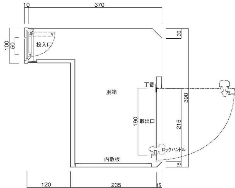
縦断面図
