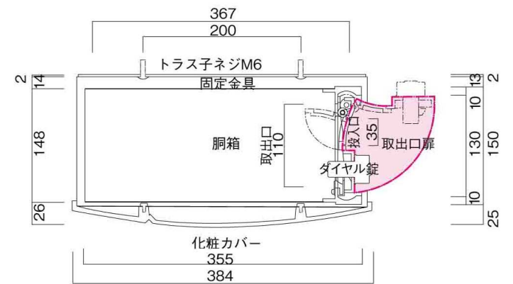
化粧カバー 355 384 横断面図
