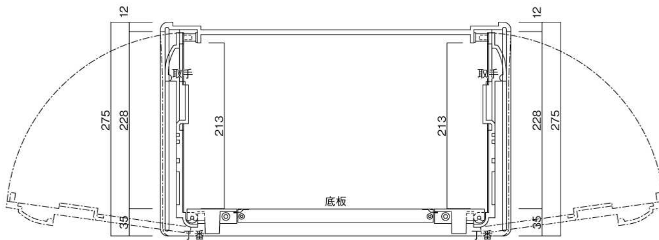
正面図
