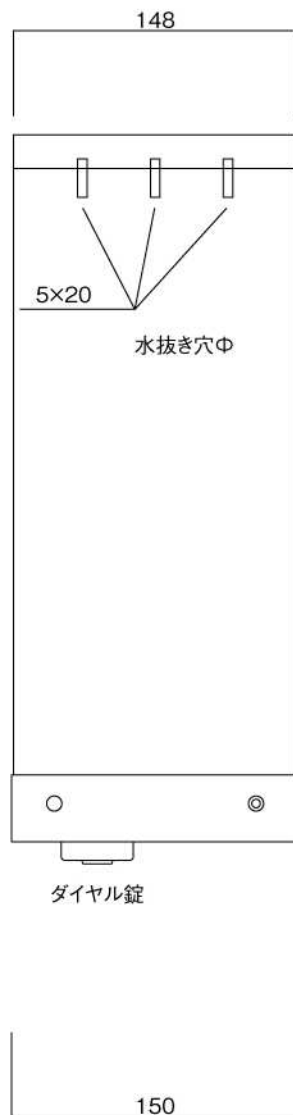
底面図
