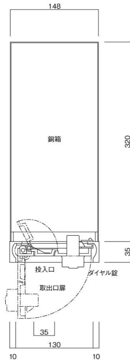
横断面図
