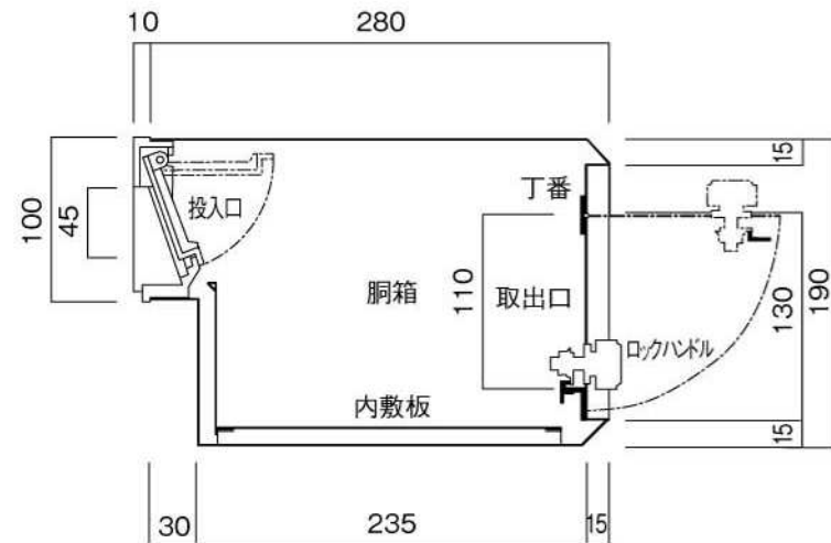
縦断面図
