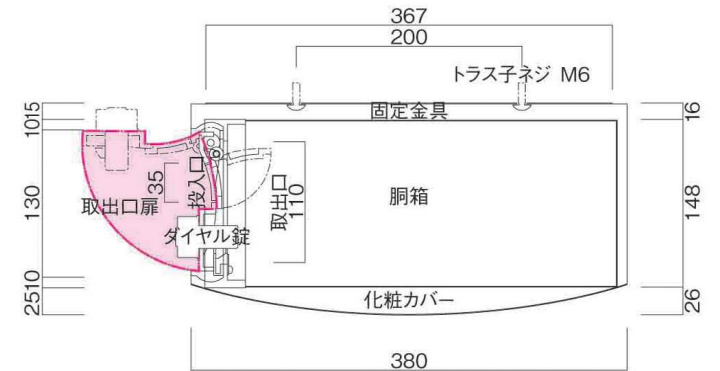
横断面図
