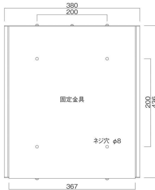
裏面図
