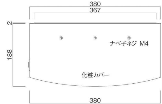
平面図
