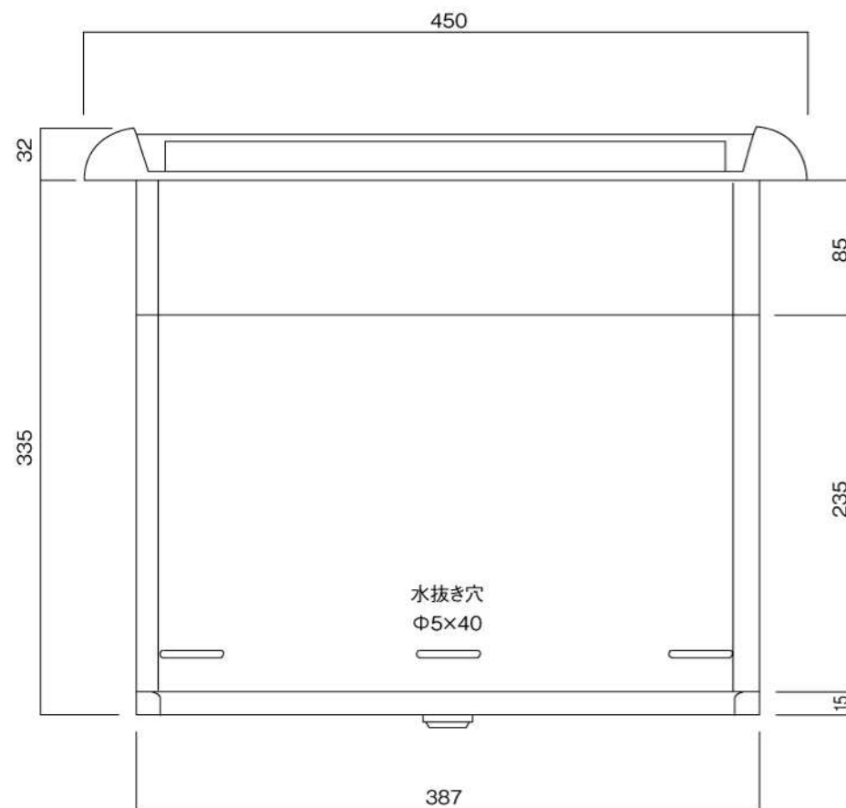
底面図
