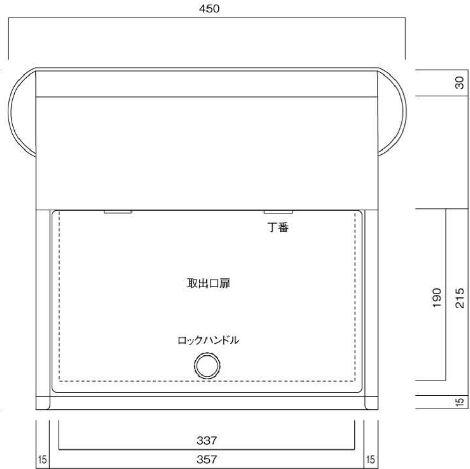
裏面図
