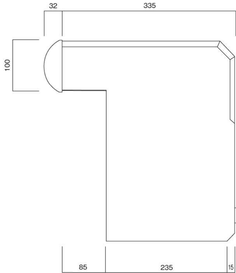
側面図
