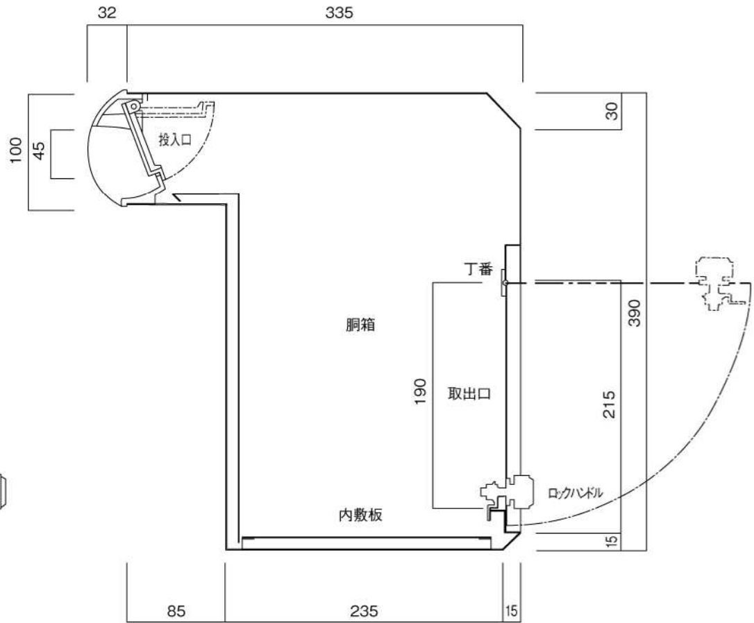
縦断面図
