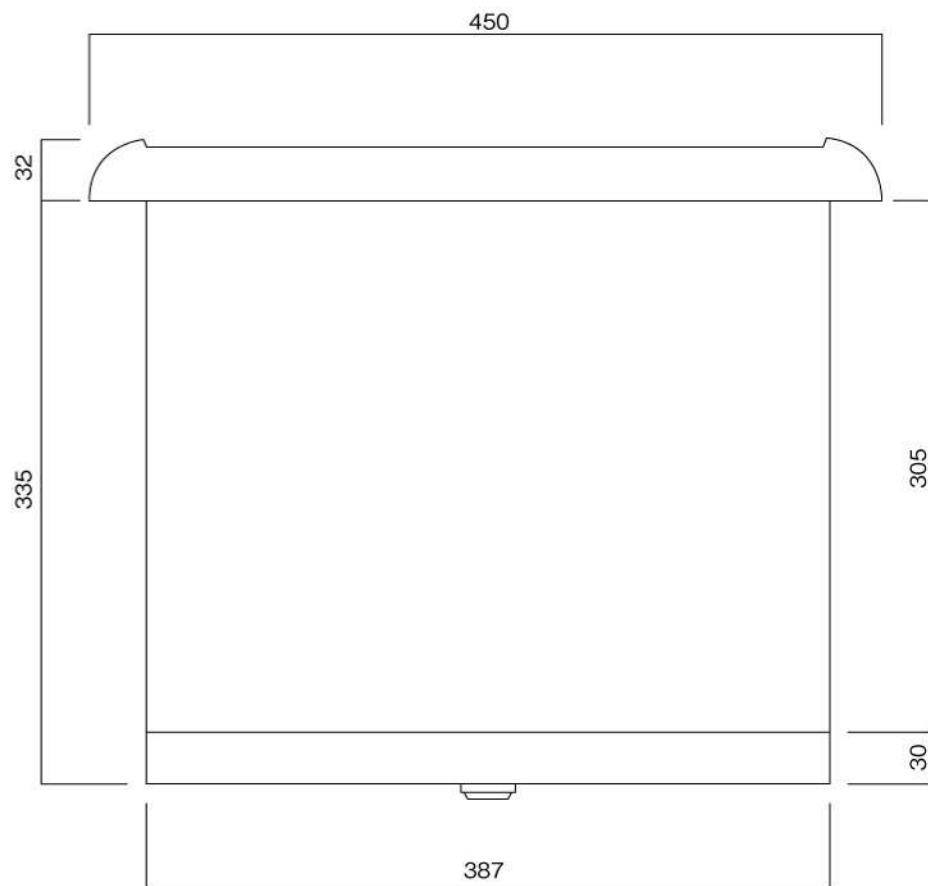
平面図
