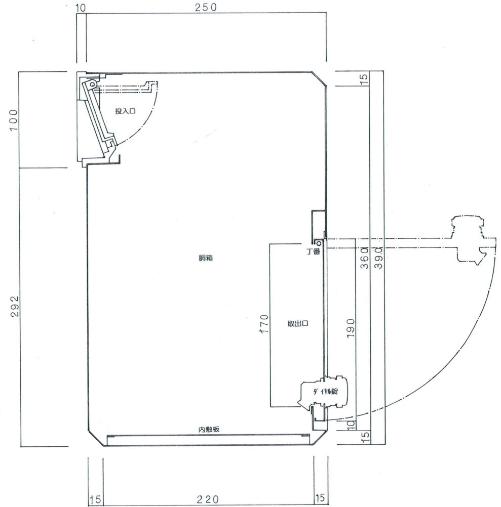
縦断面図
