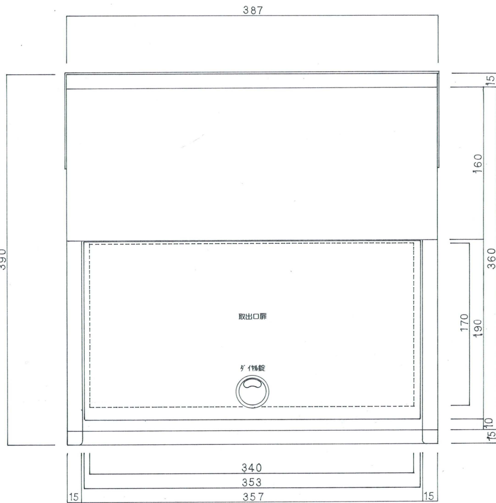
裏面図
