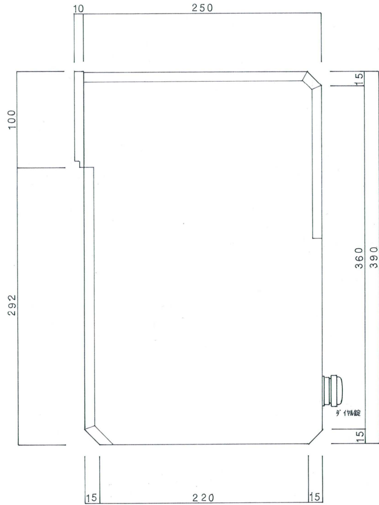
側面図
