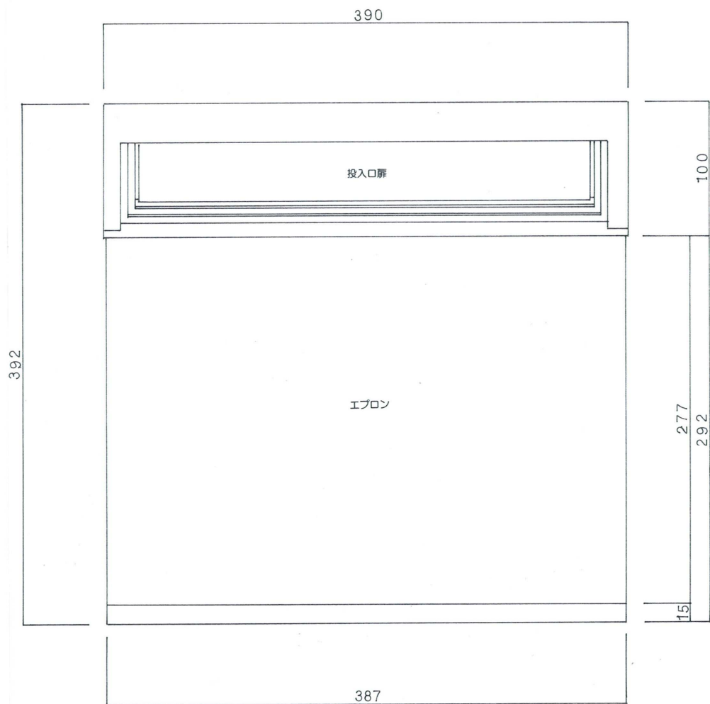
正面図
