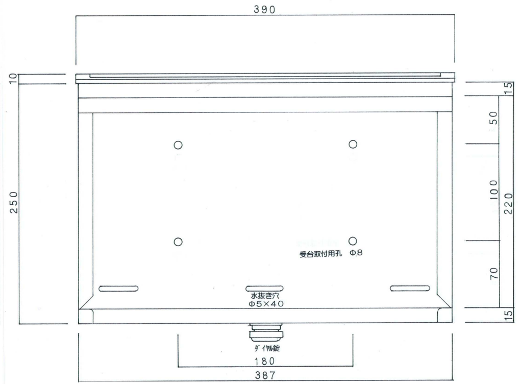
底面図
