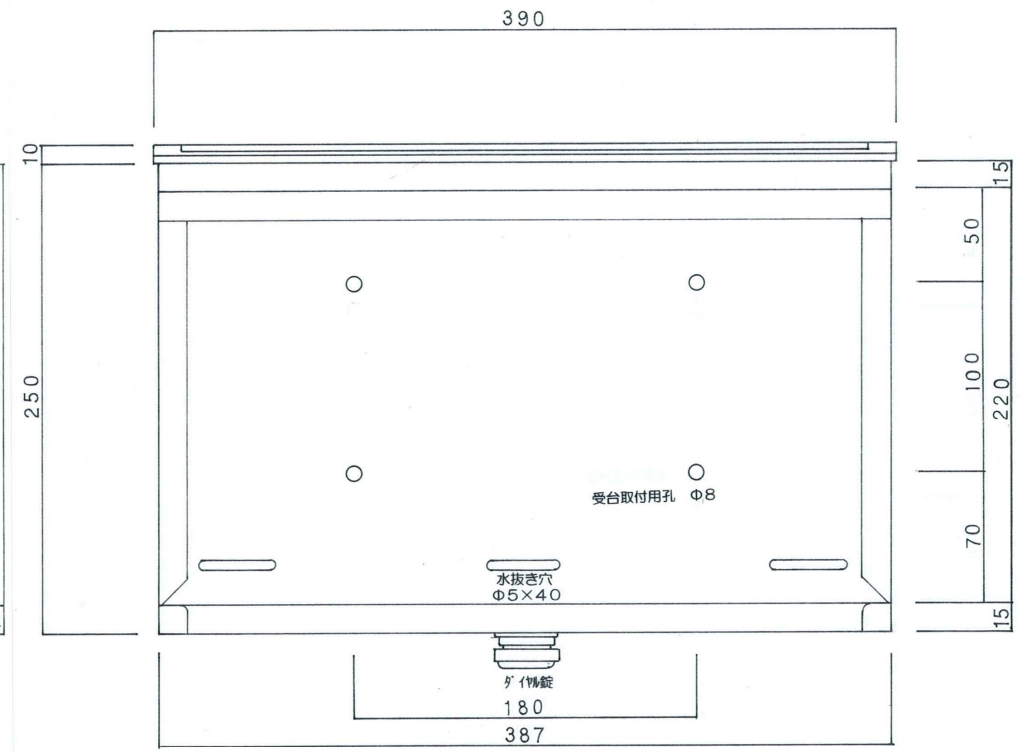
底面図
