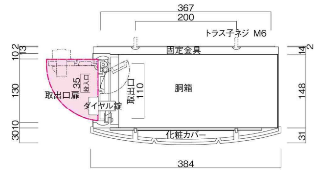
横断面図
