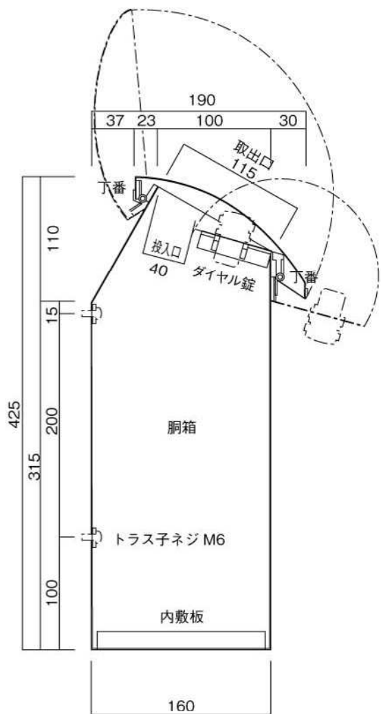
縦断面図
