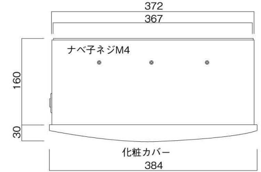
平面図
