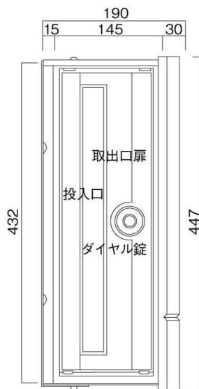
左側面図
