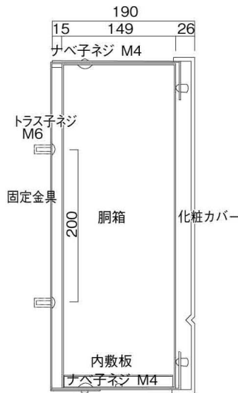
縦断面図
