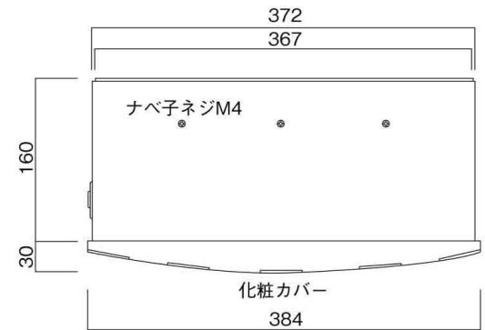
平面図
