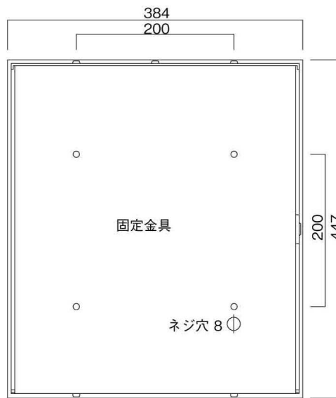
裏面図
