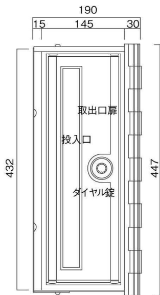
左側面図
