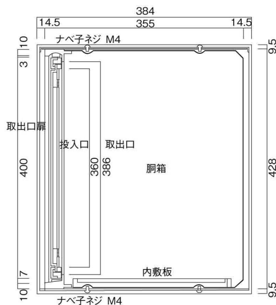
縦断面図
