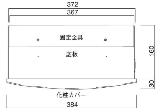
化粧カバー 384 底面図
