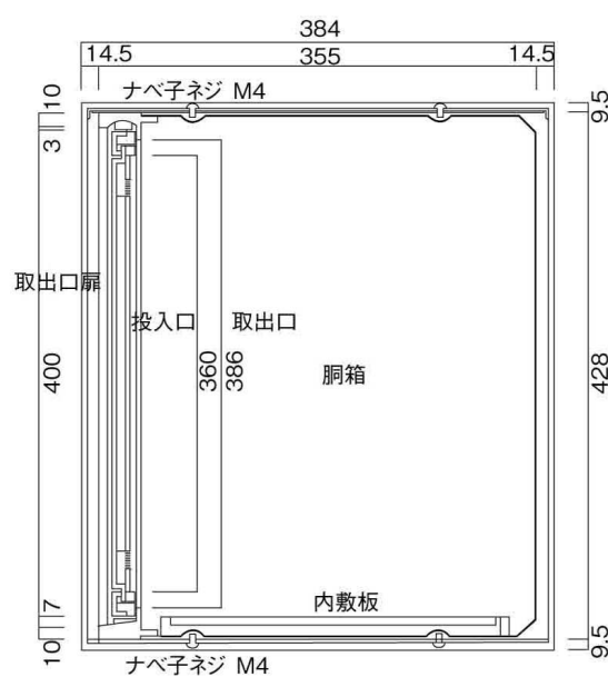
縦断面図
