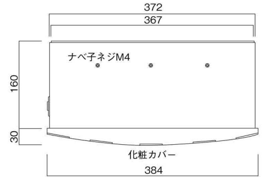
化粧カバー 384 平面図
