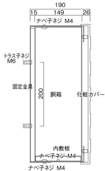
縦断面図
