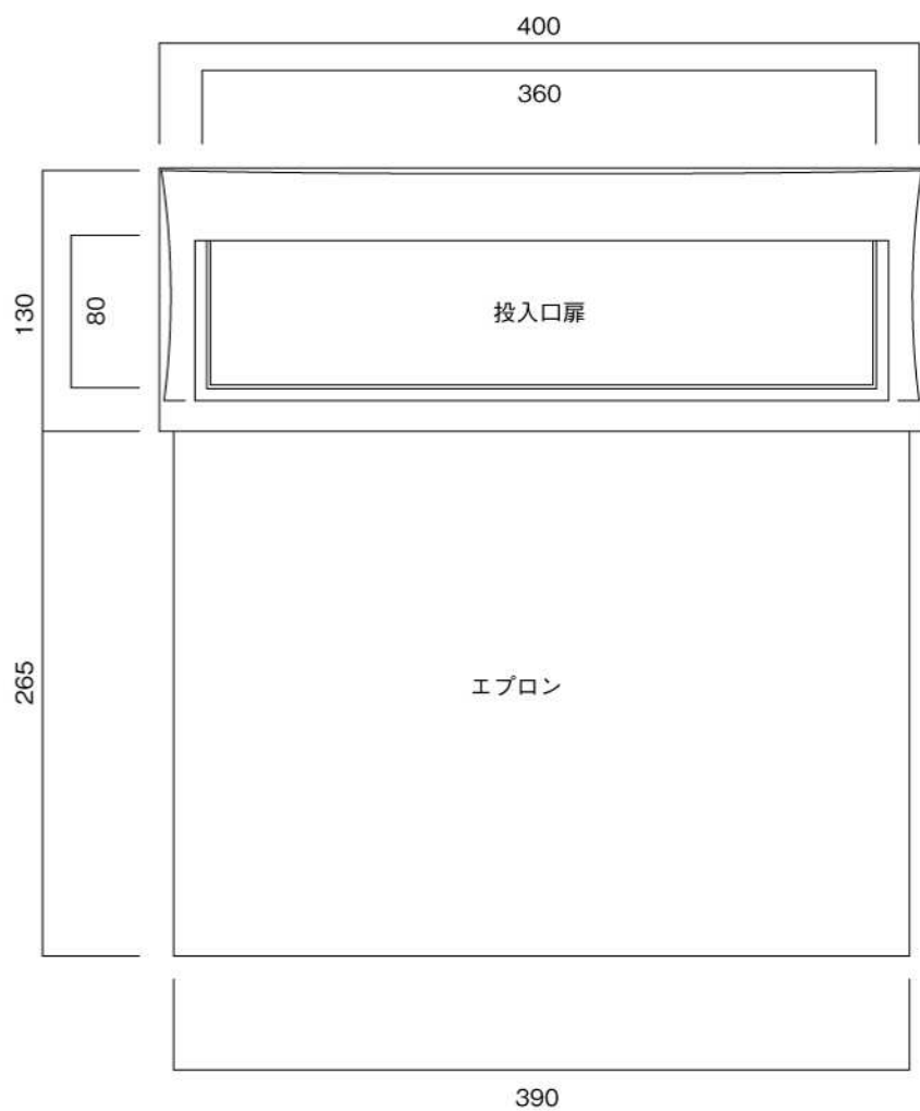
正面図
