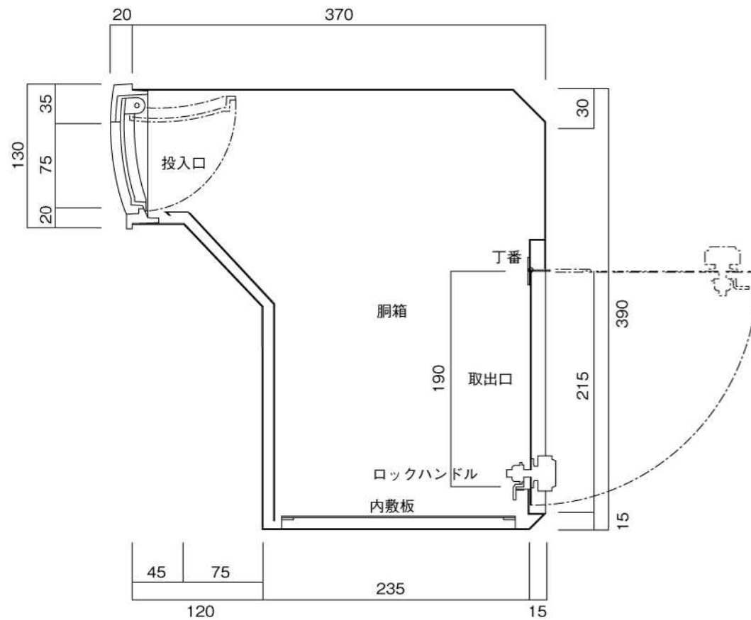
縦断面図
