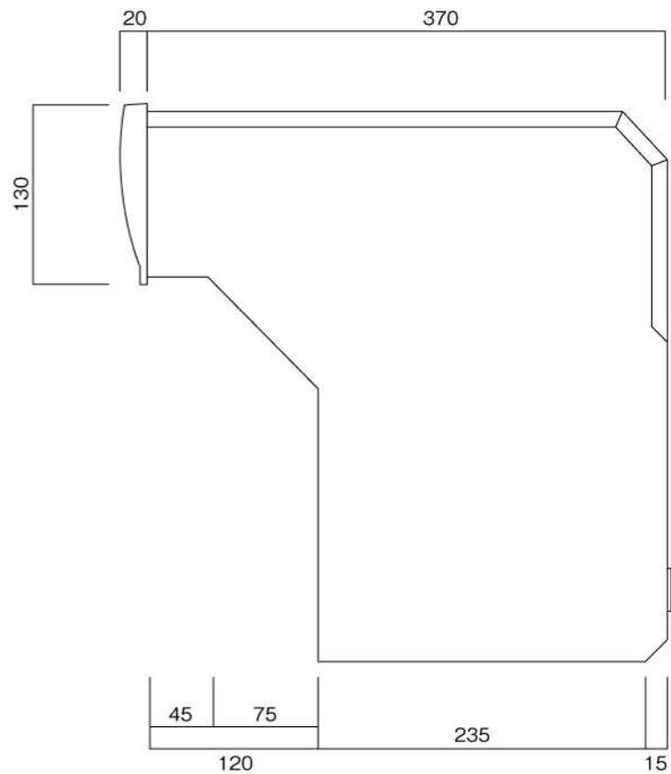
側面図
