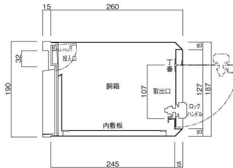
縦断面図
