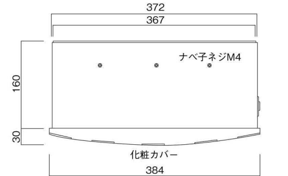
化粧カバー 384 平面図
