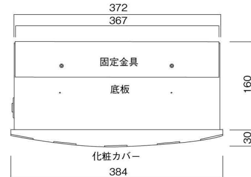
化粧カバー 384 底面図
