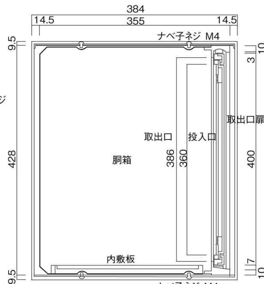
縦断面図
