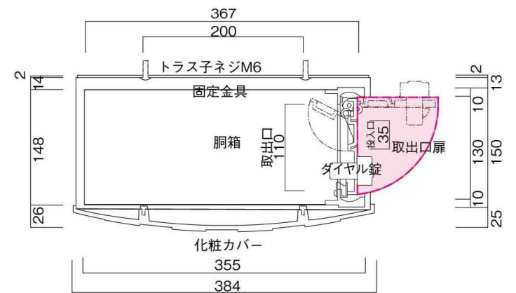
化粧カバー 355 384 横断面図
