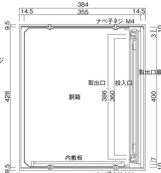
縦断面図
