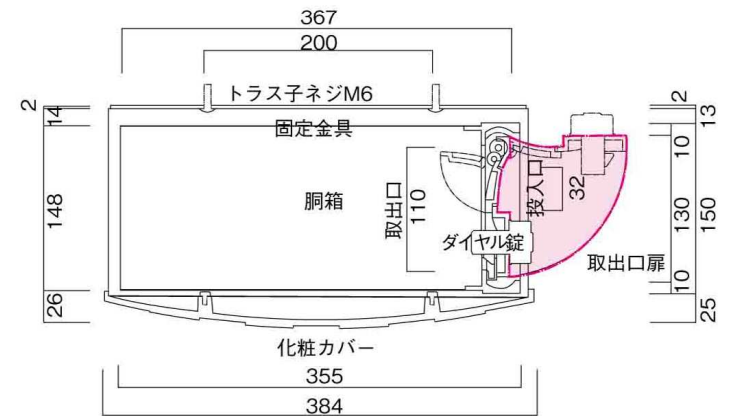
横断面図
