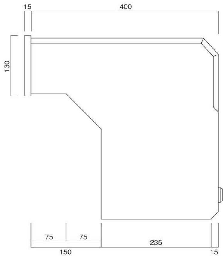
側面図
