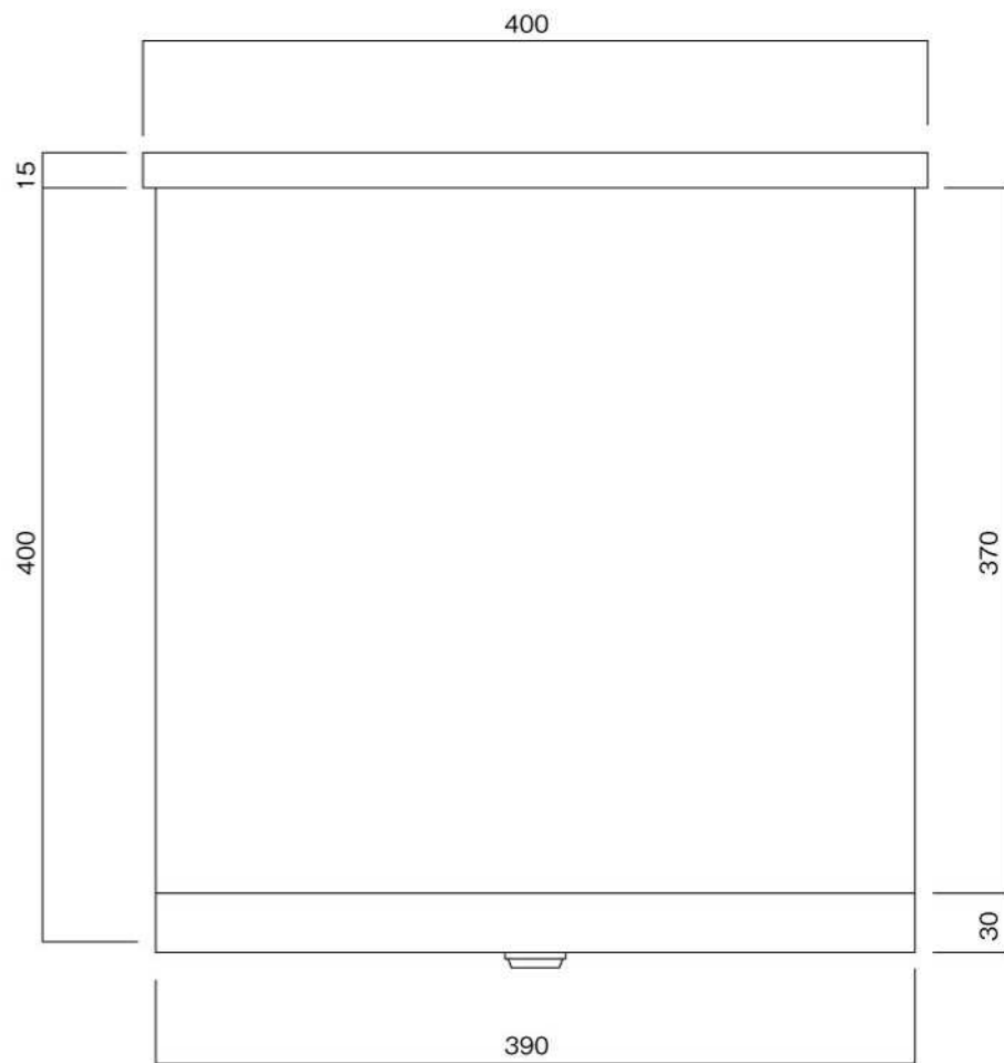
平面図
