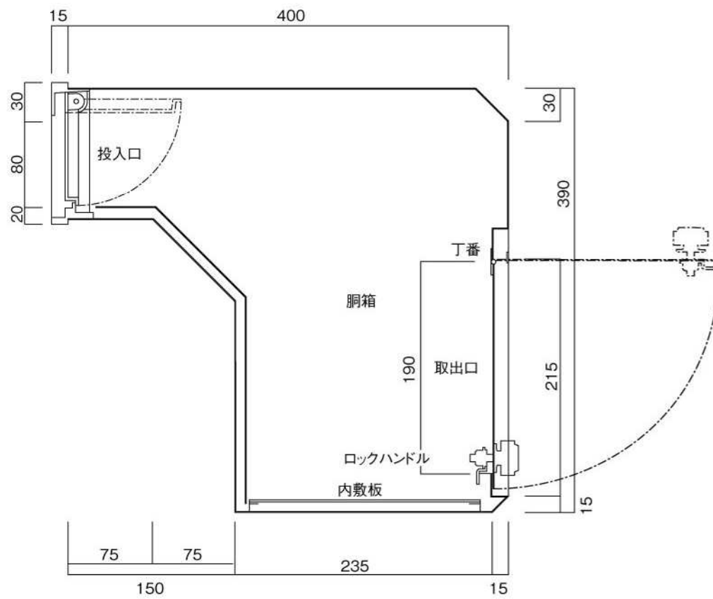
縦断面図
