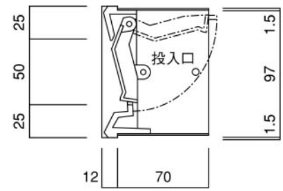
側面図
