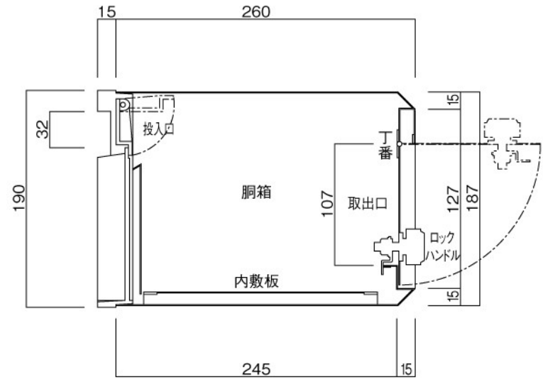
縦断面図
