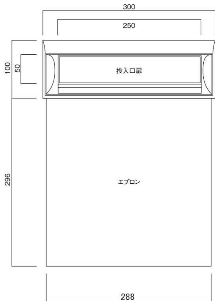
正面図
