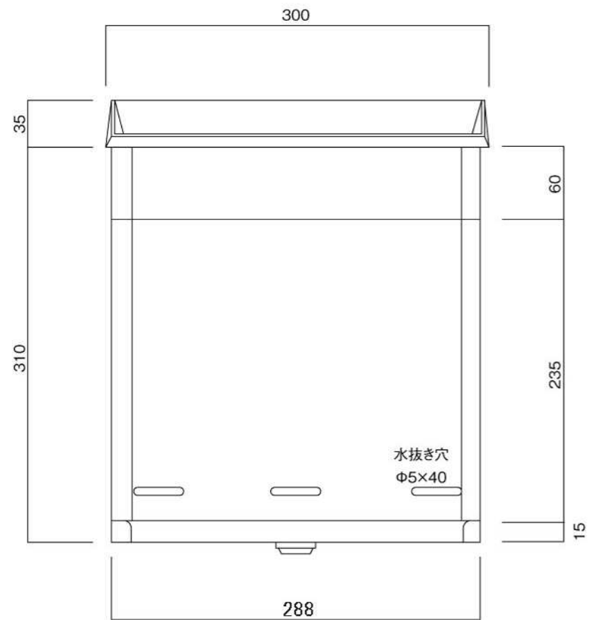
底面図
