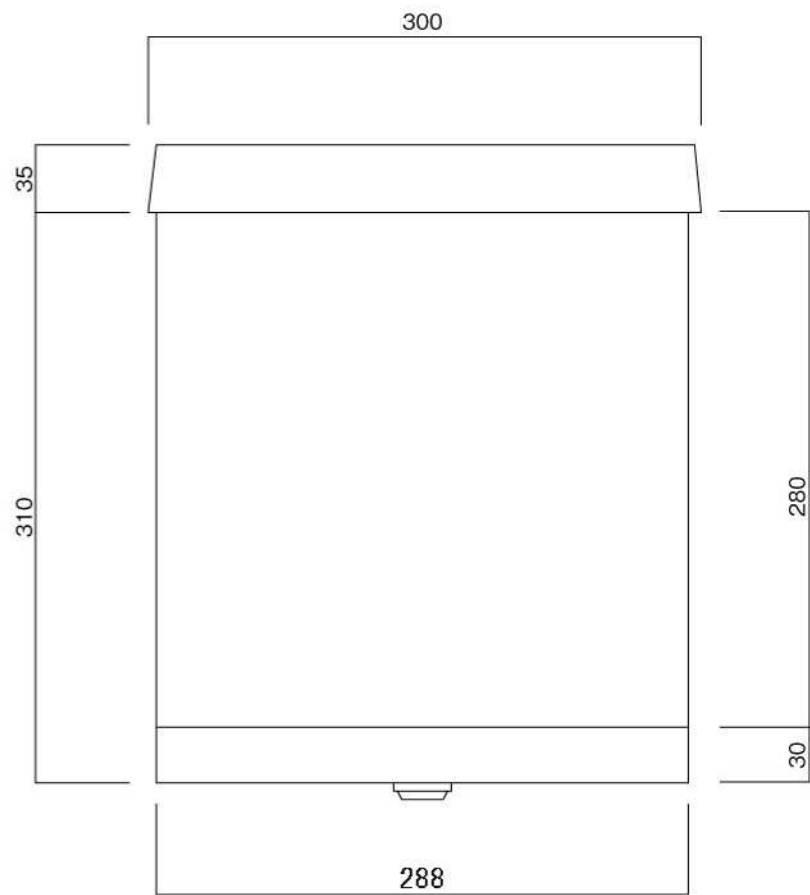
平面図
