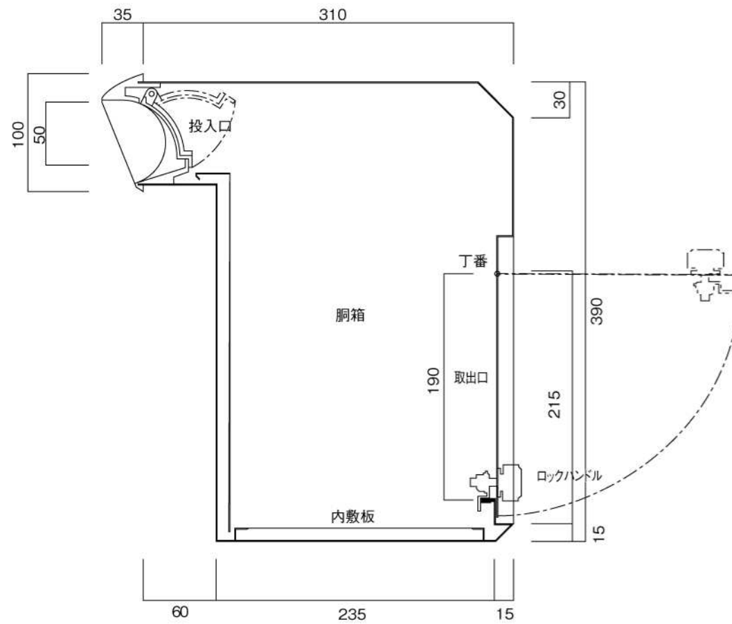
縦断面図
