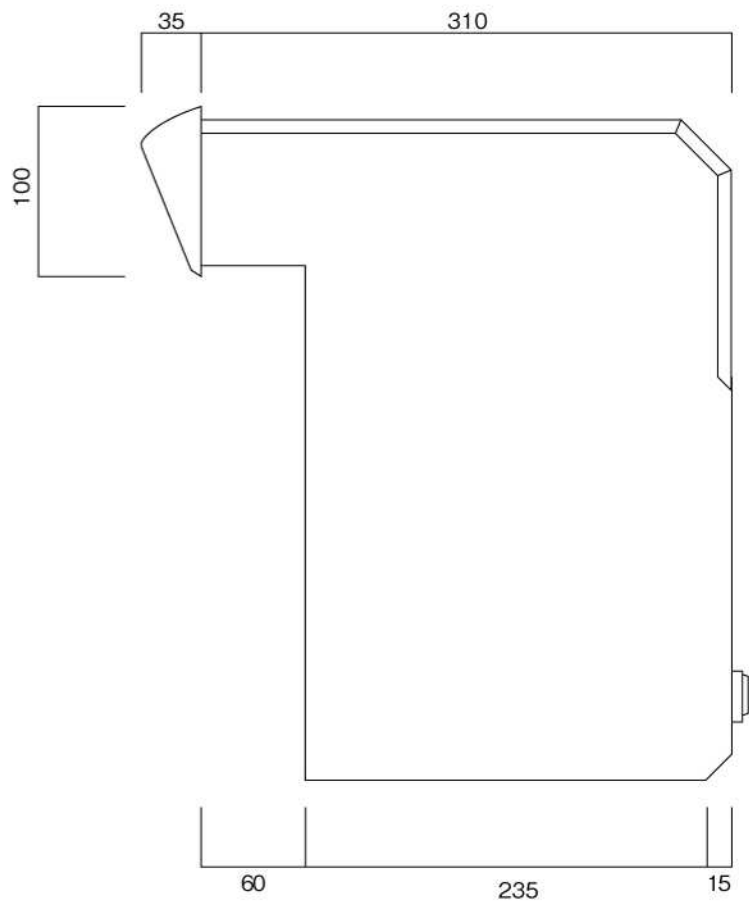
側面図
