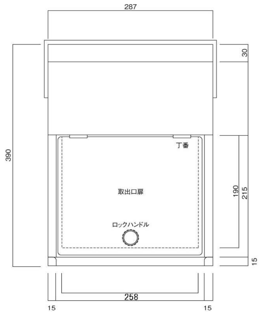
裏面図
