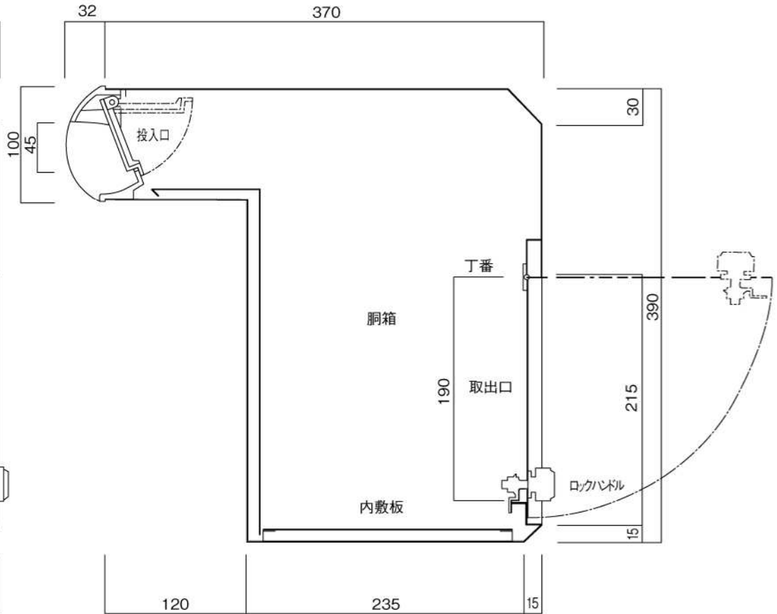
縦断面図
