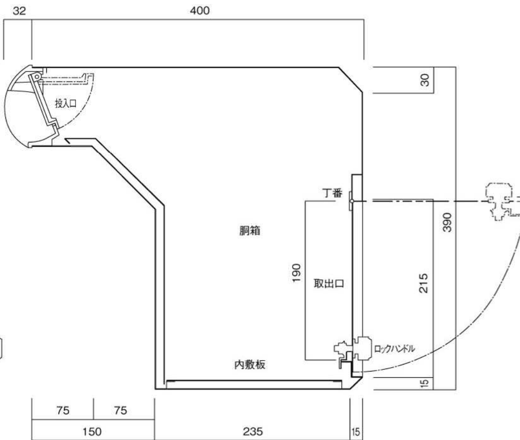
縦断面図
