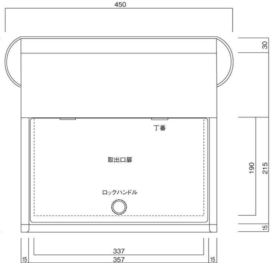
裏面図
