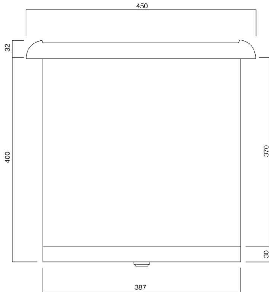
平面図
