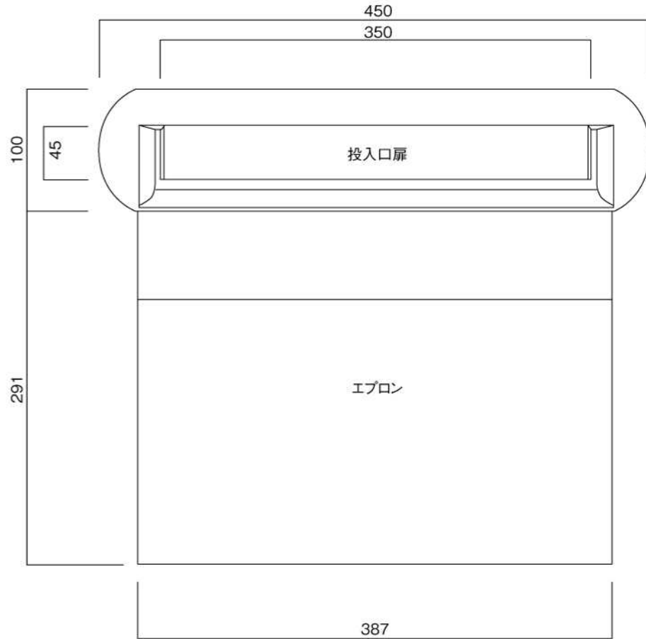
正面図
