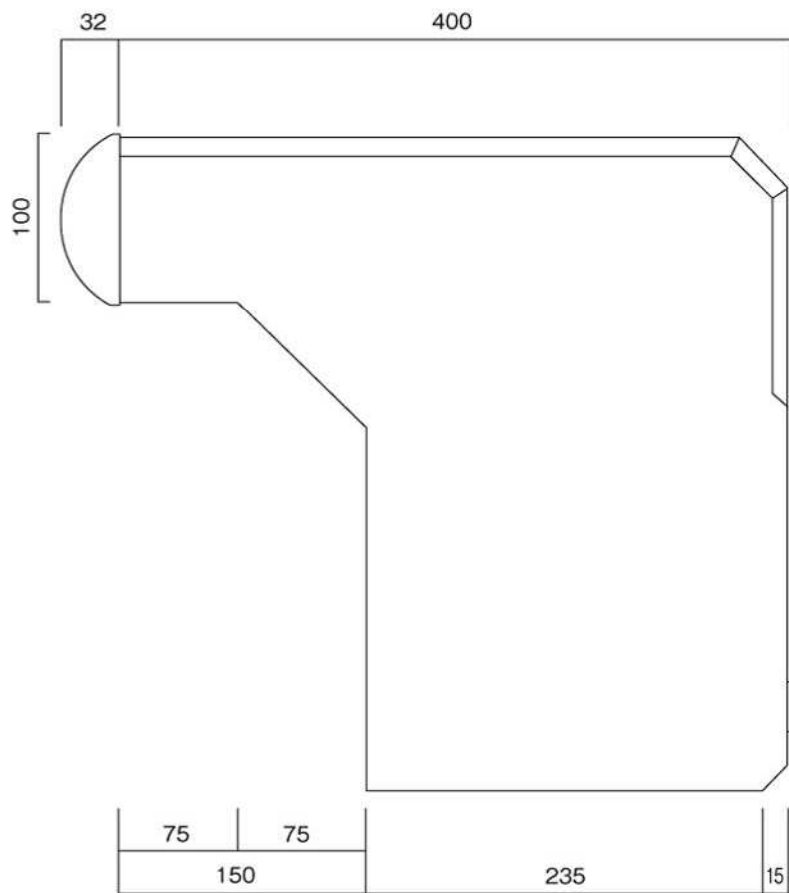
側面図
