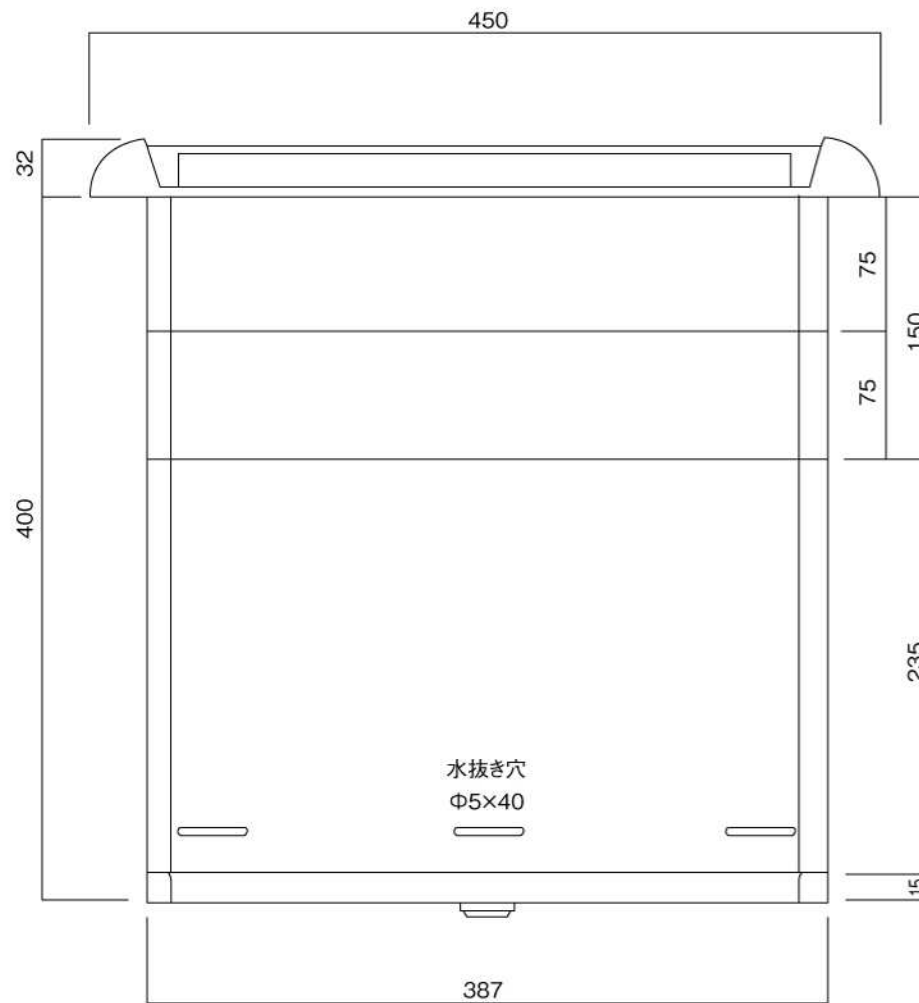
底面図
