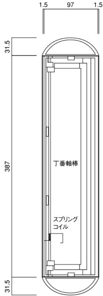
裏面図
