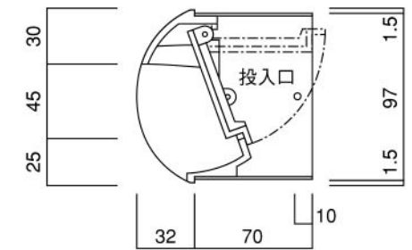
縦断面図
