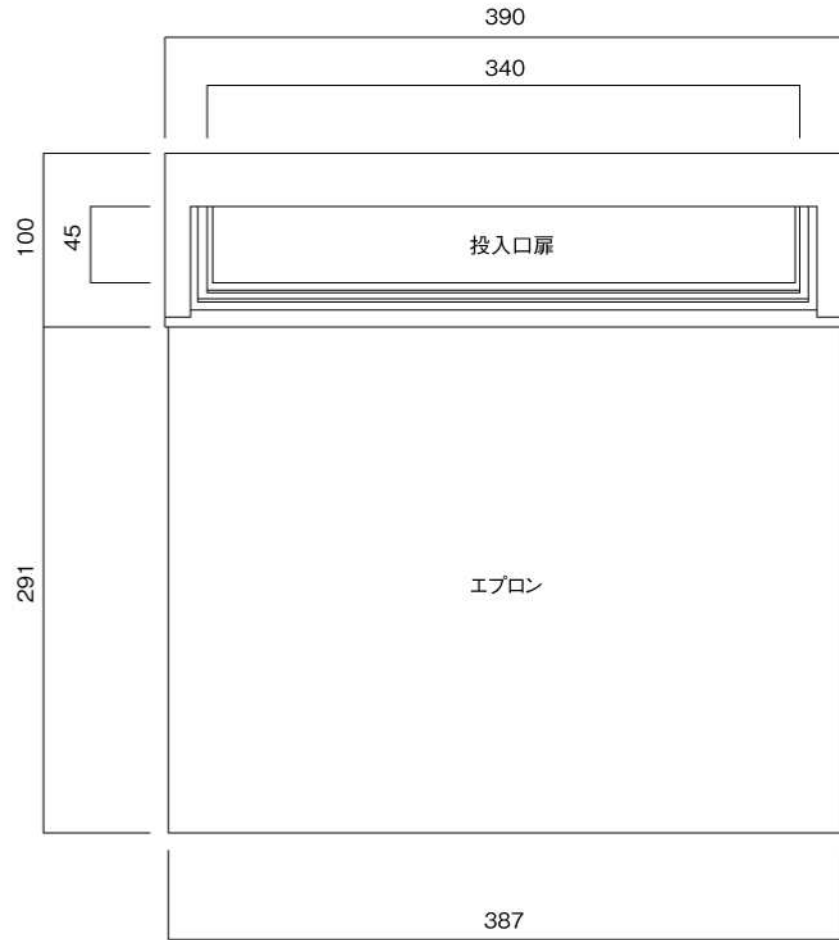
正面図
