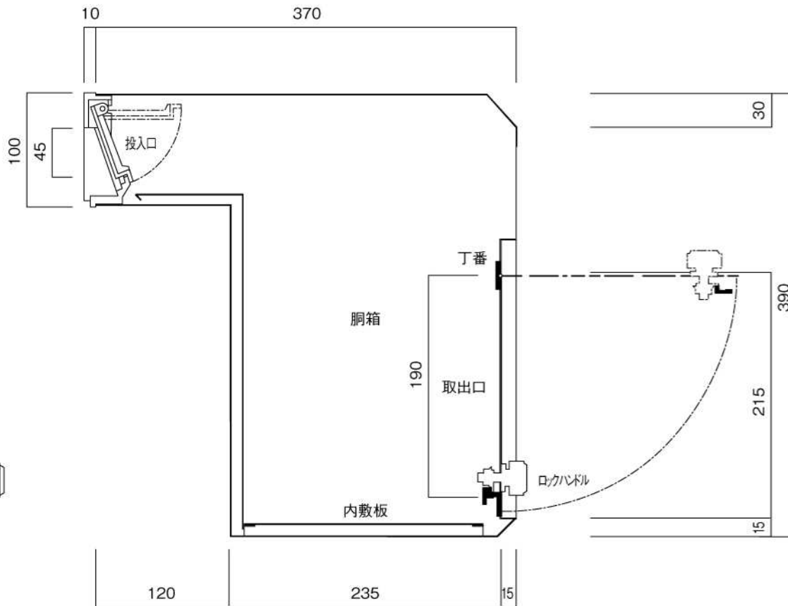
縦断面図
