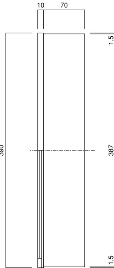
平面図
