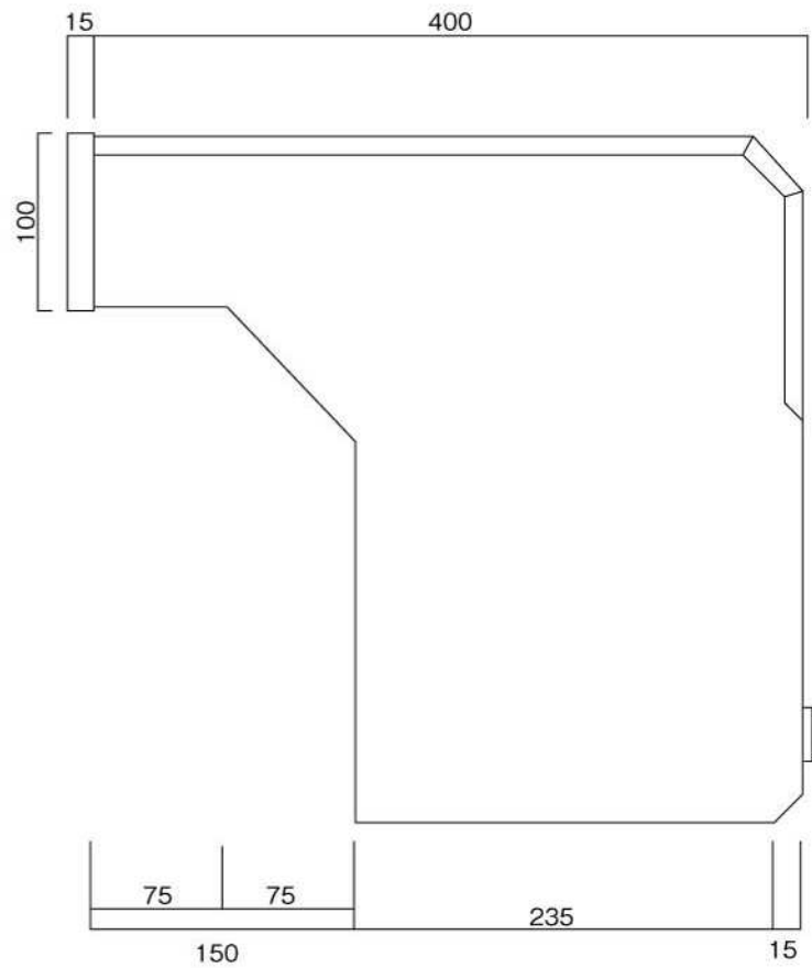
側面図
