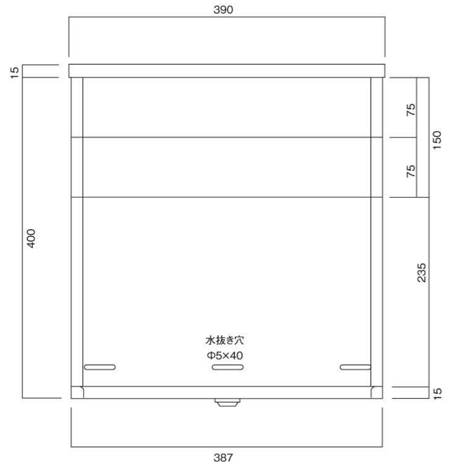
底面図
