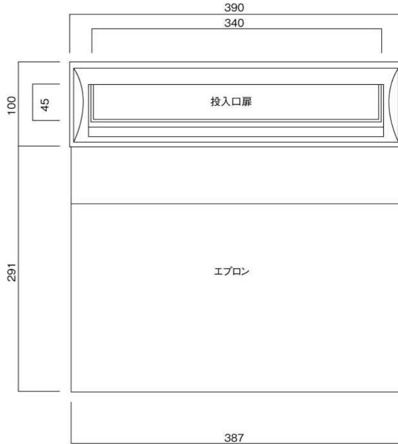
正面図
