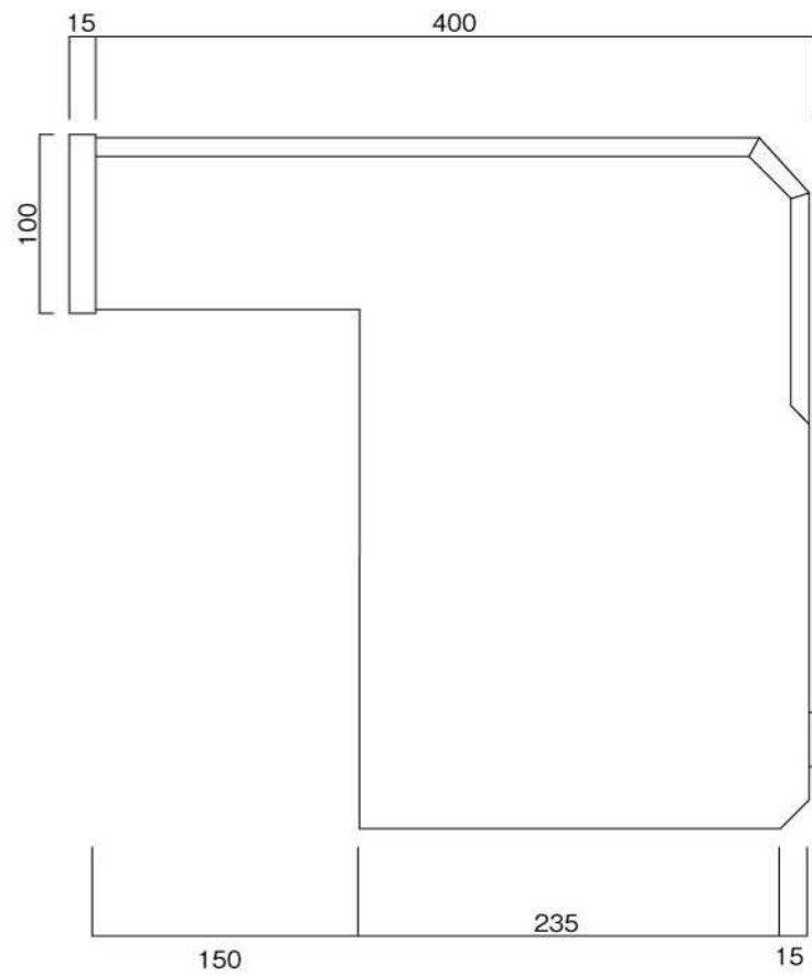
側面図
