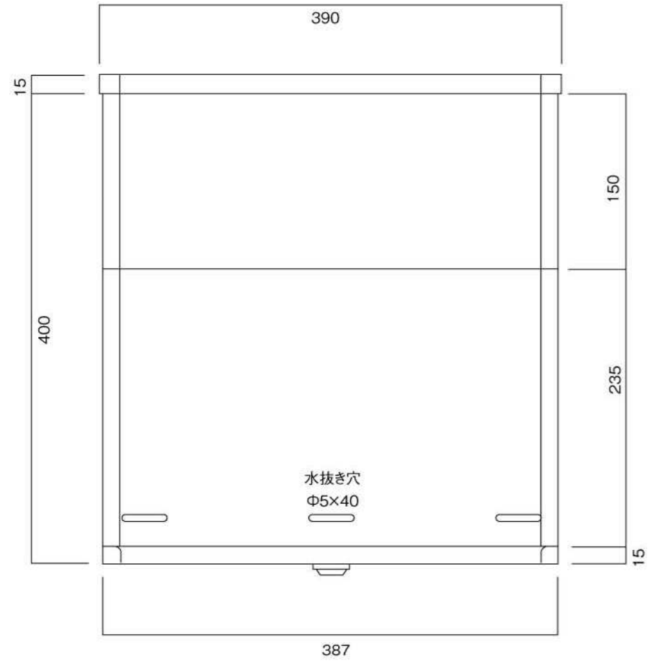
底面図
