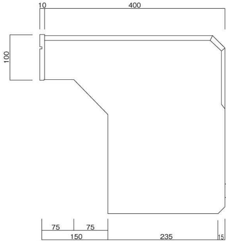
側面図
