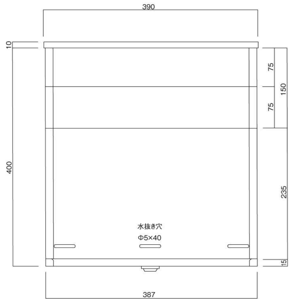
底面図
