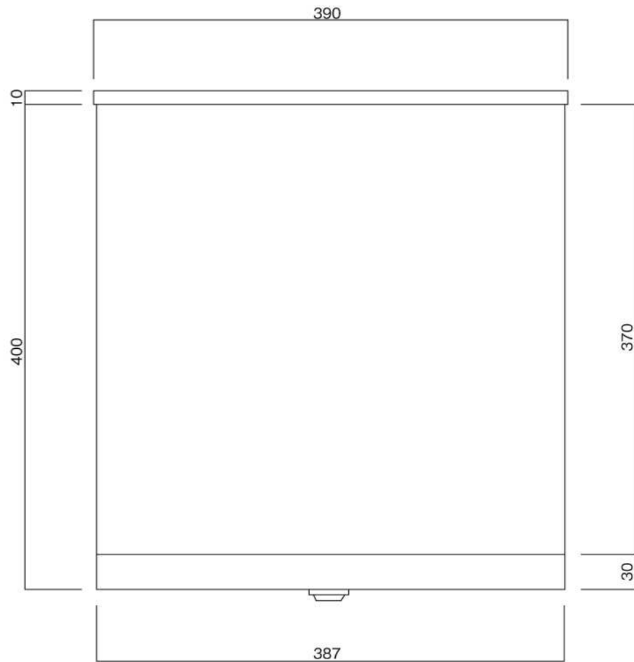
平面図
