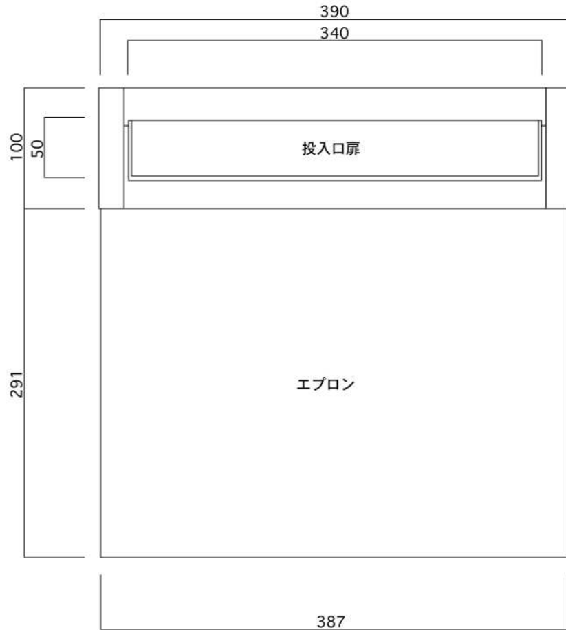
平面図
