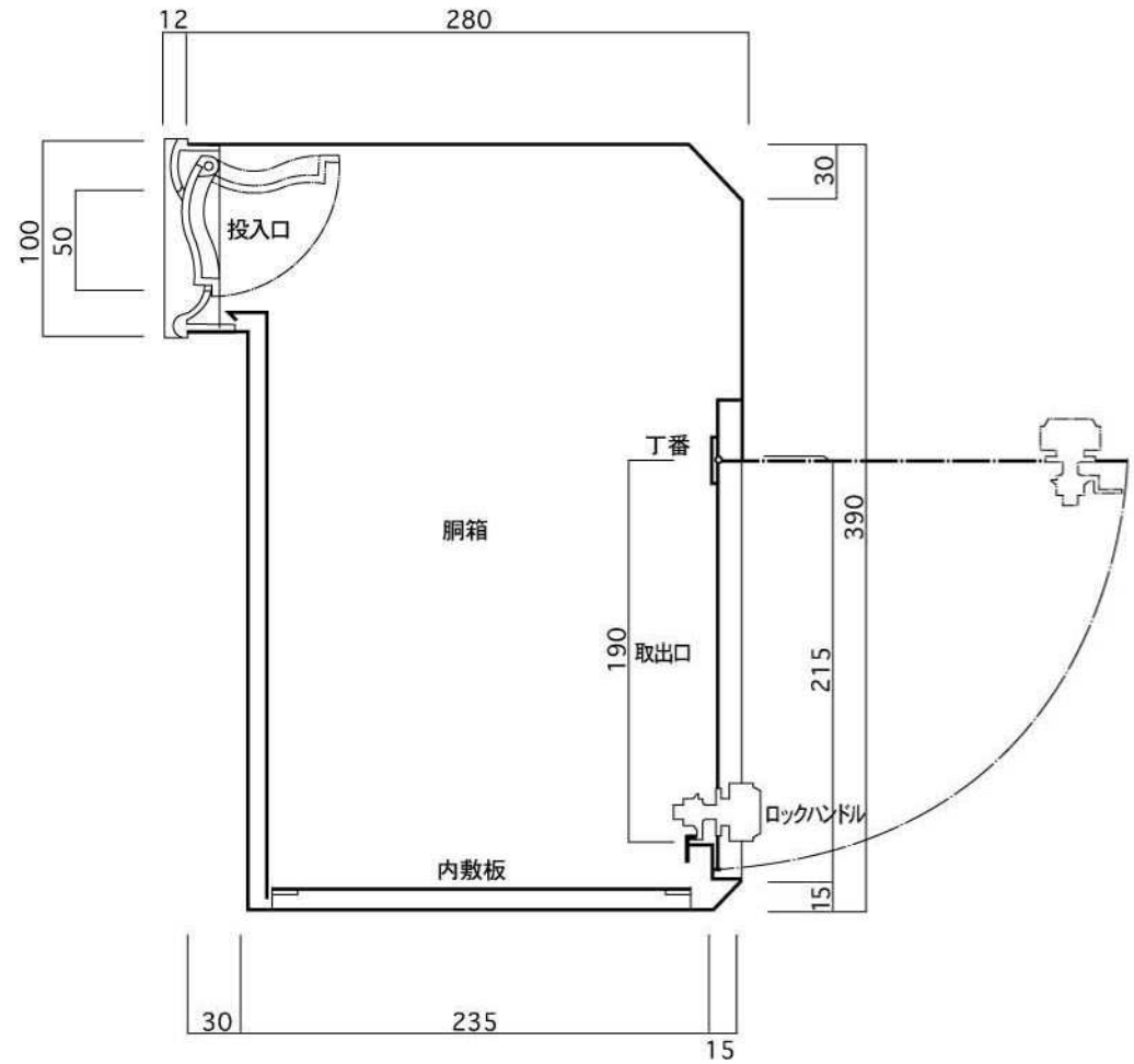
縦断面図
