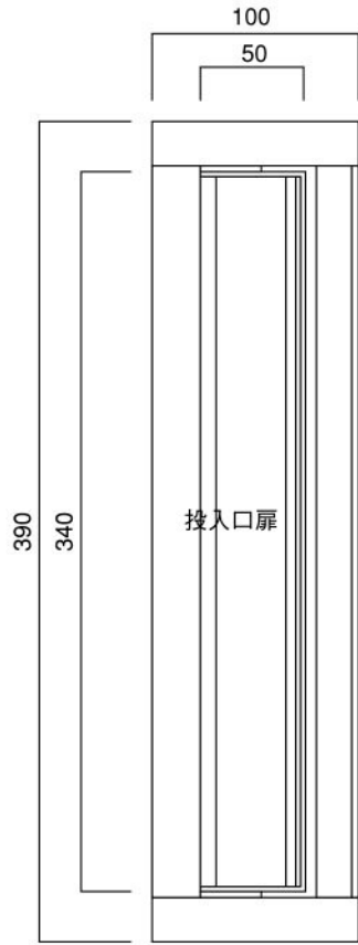
正面図
