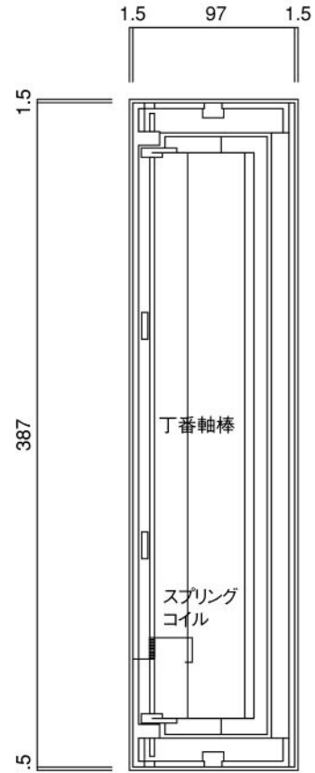
裏面図
