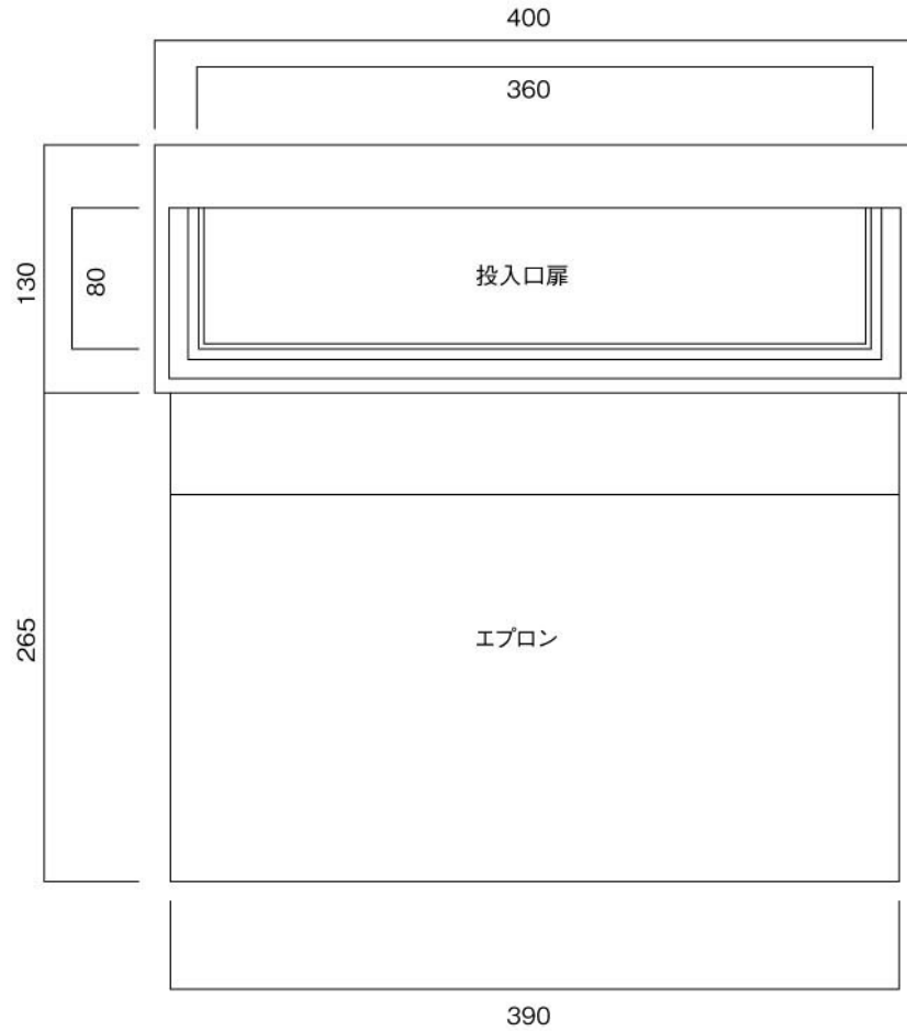
正面図
