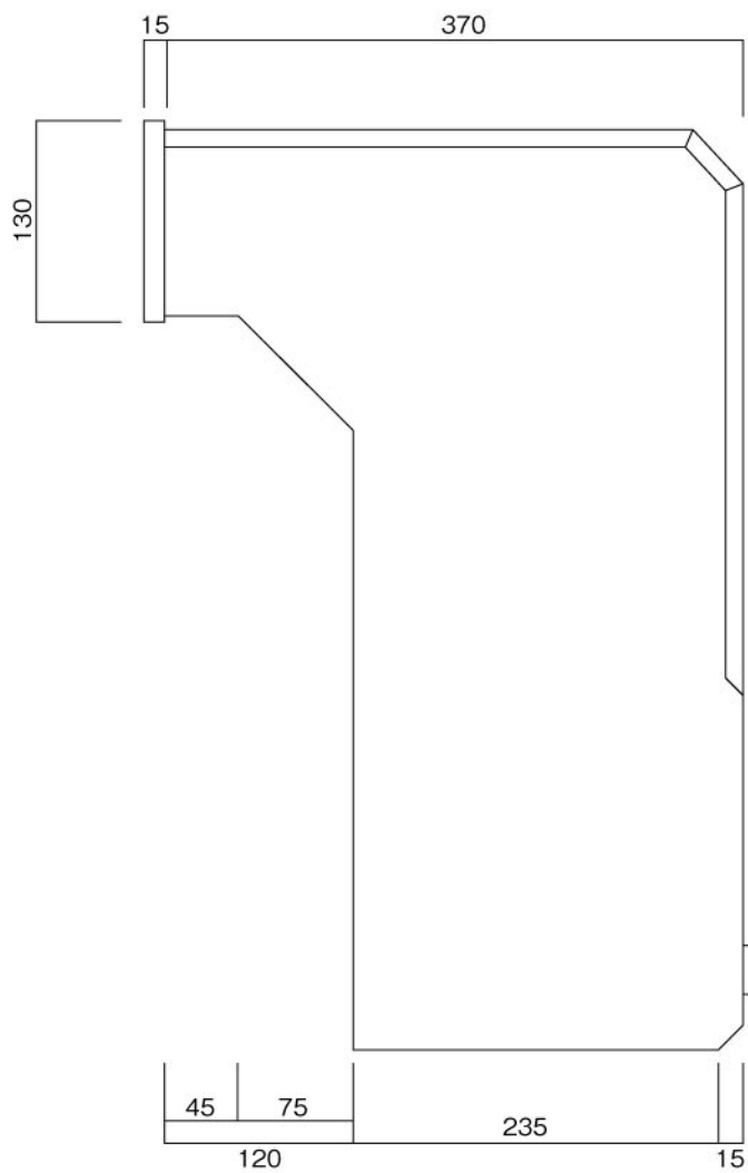
側面図
