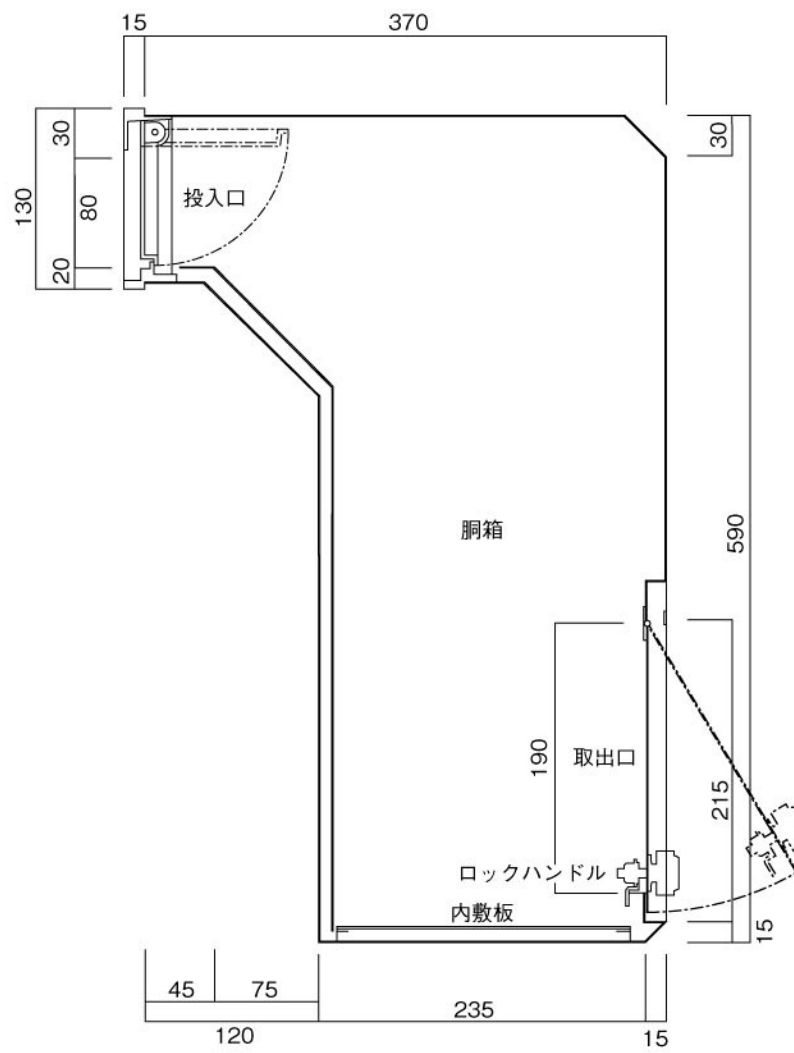
縦断面図
