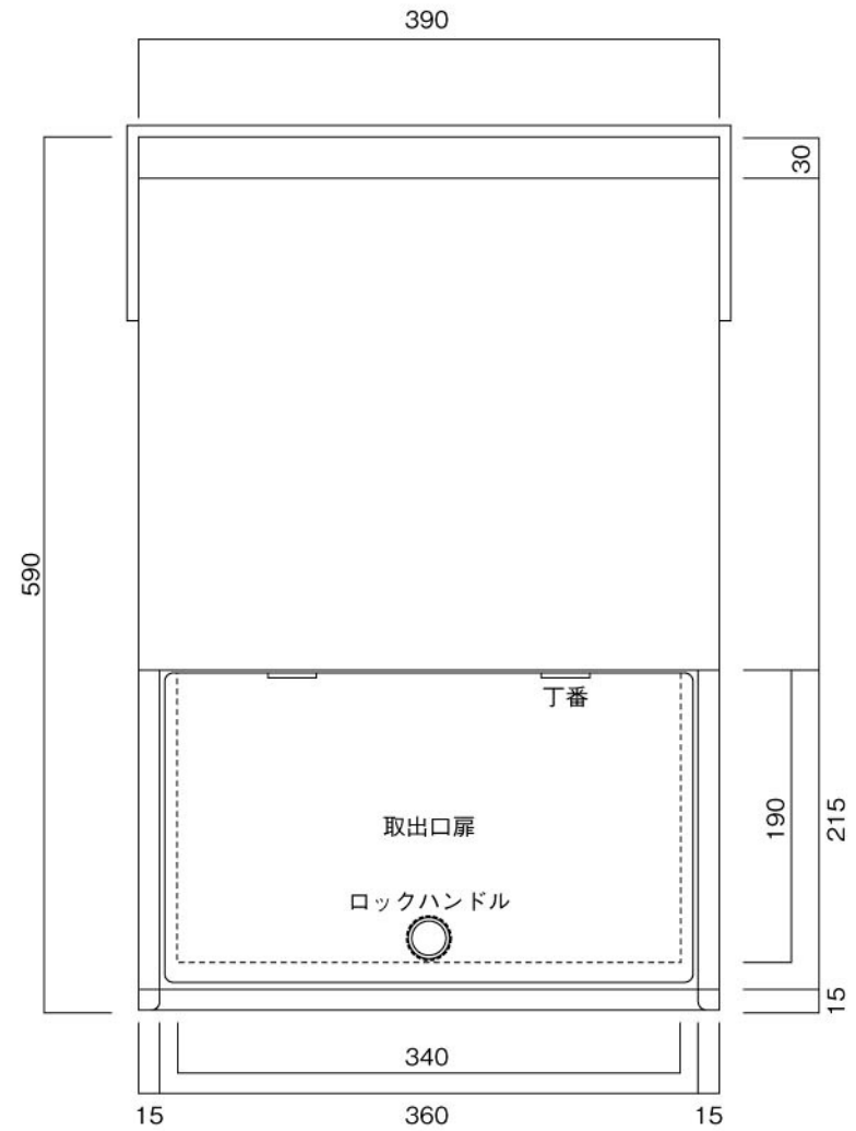
裏面図
