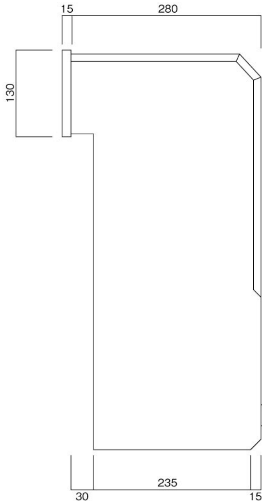
側面図
