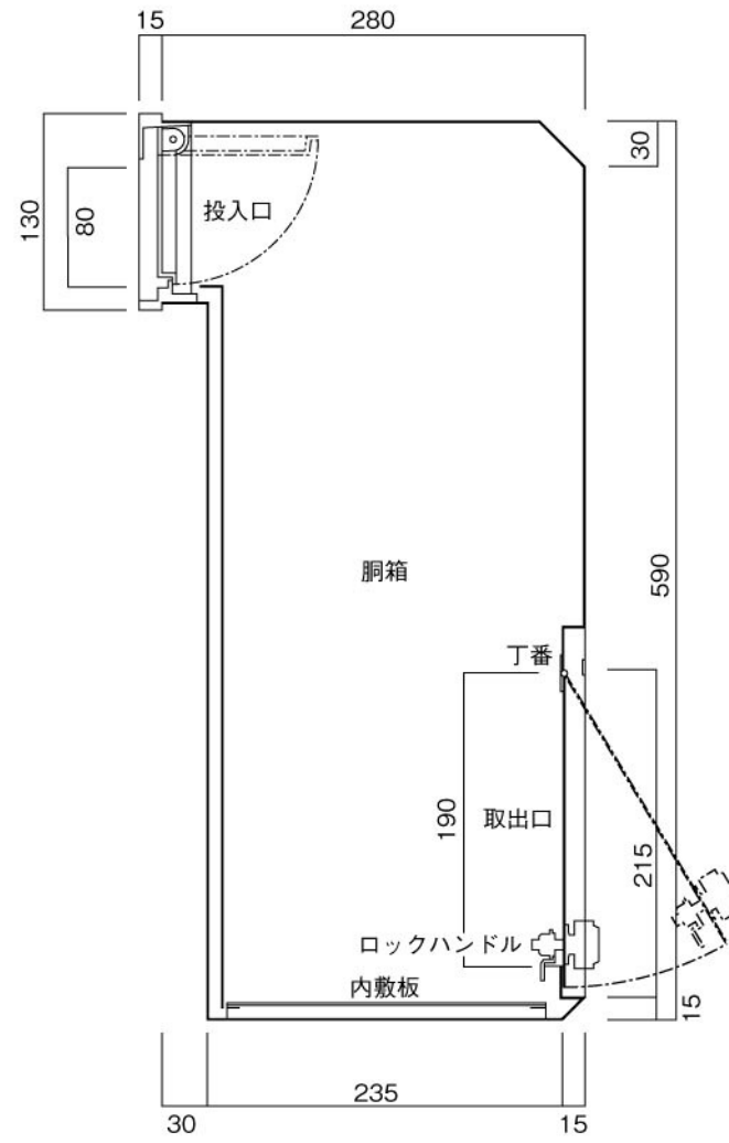
縦断面図
