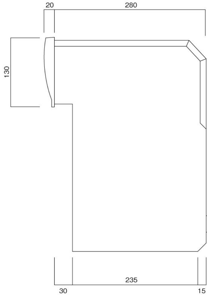
側面図
