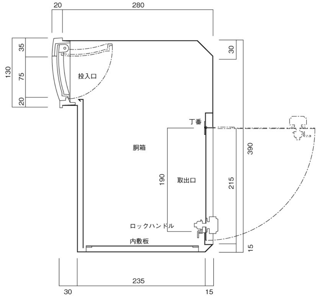
縦断面図
