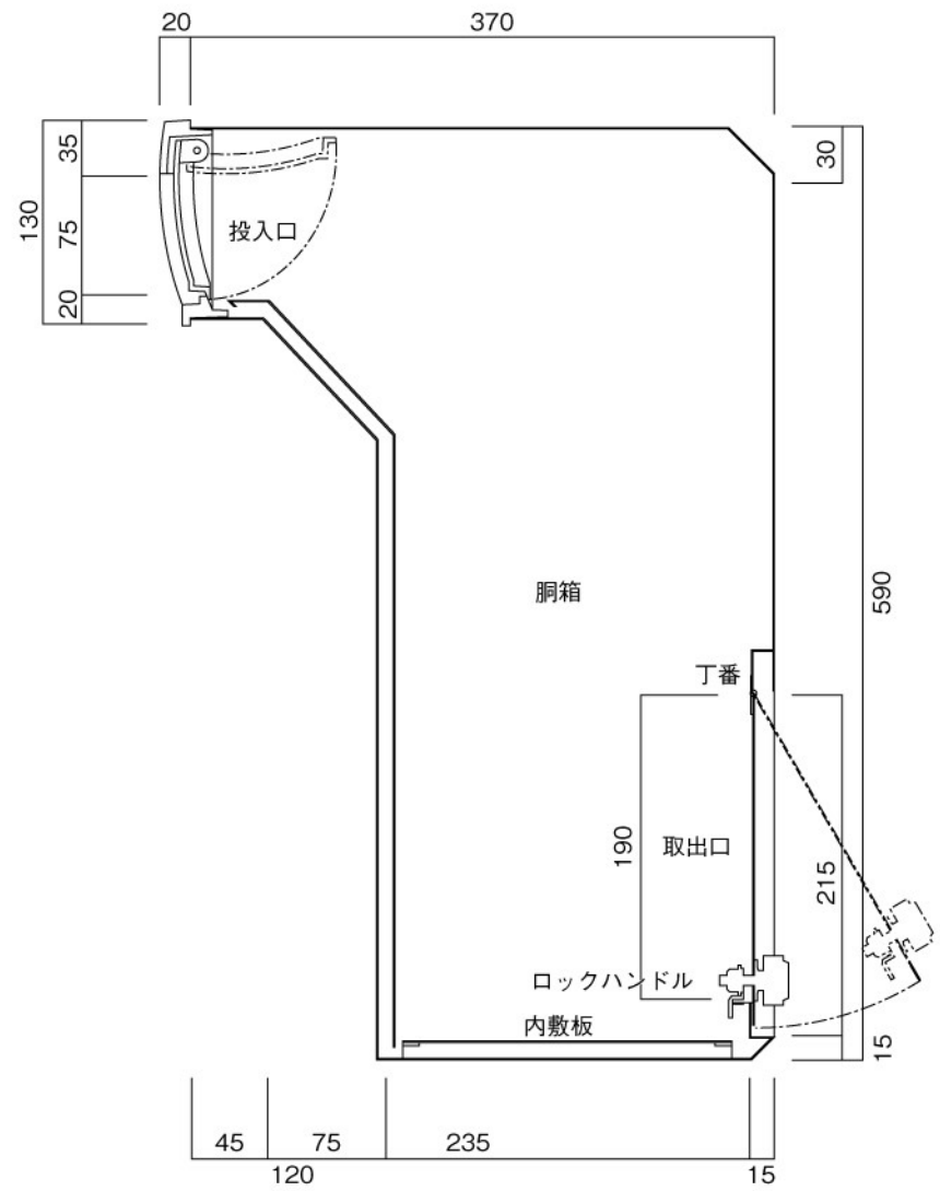
縦断面図
