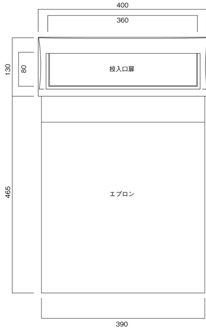
正面図
