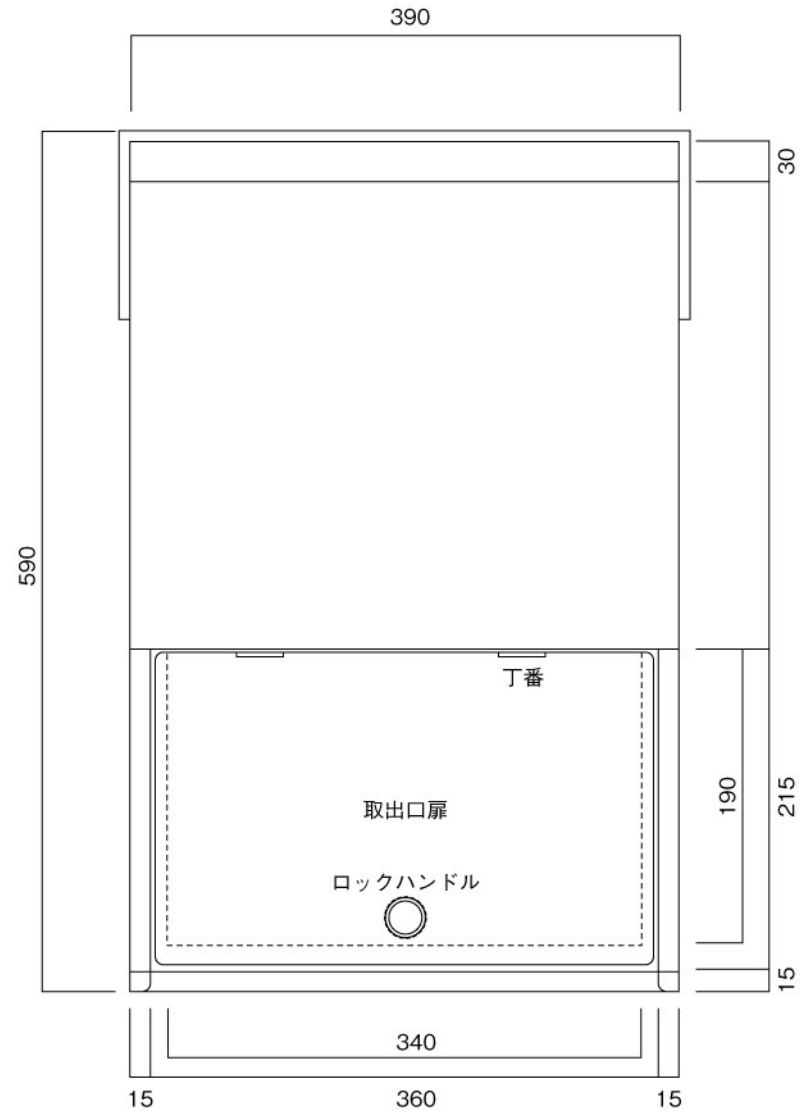
裏面図
