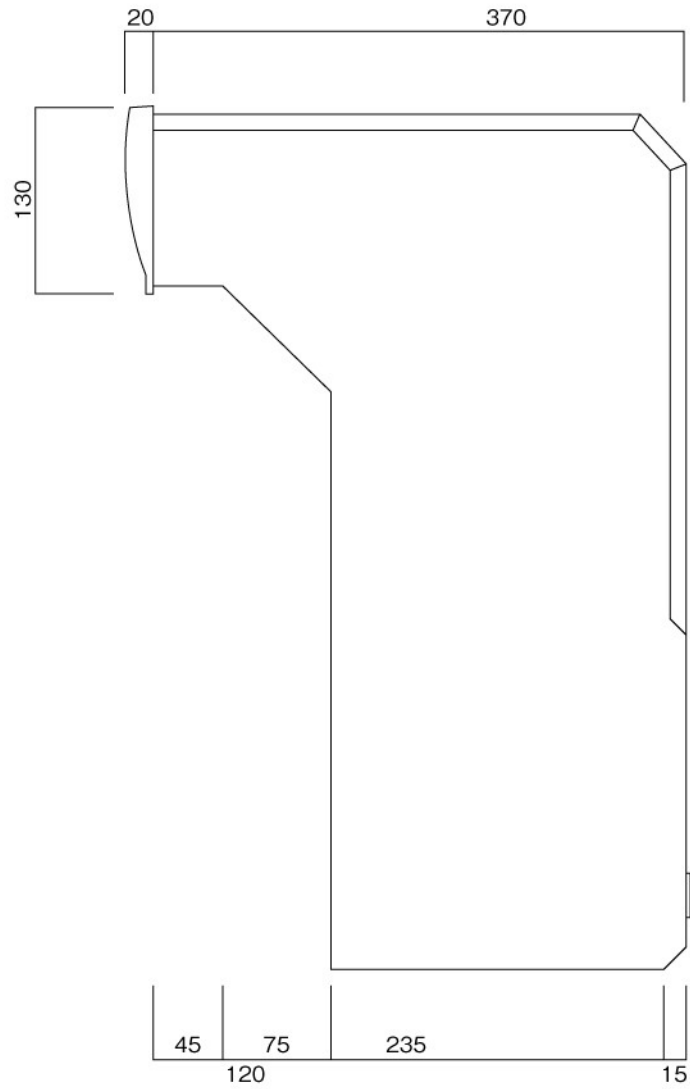
側面図
