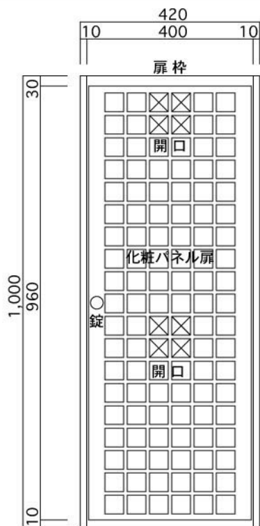
正面図
