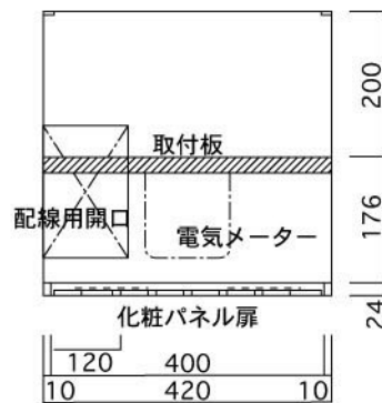
横断面図
