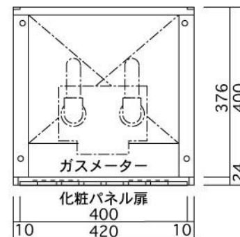
横断面図
