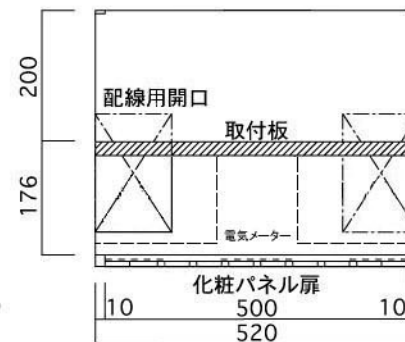
横断面図
