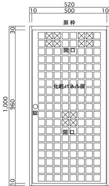
正面図
