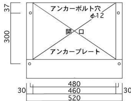
底面図
