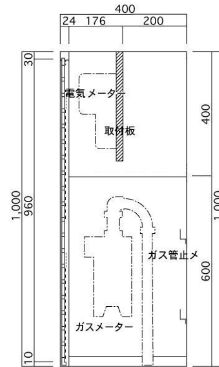
側面図
