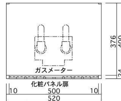
横断面図
