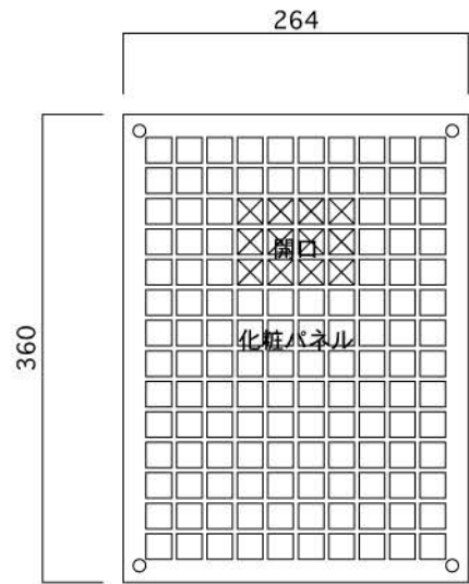
正面図
