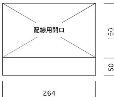
底面図
