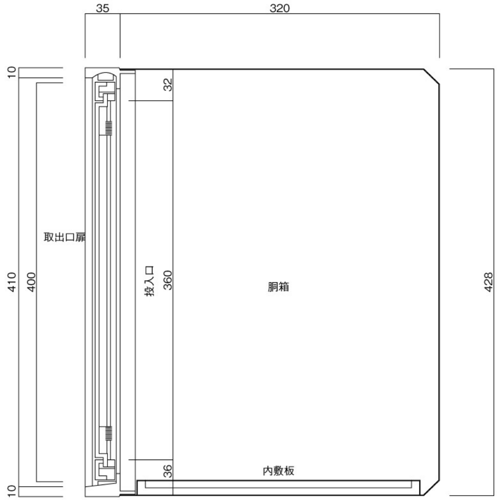
縦断面図
