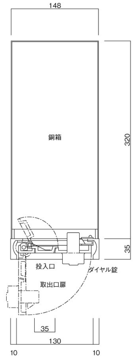
横断面図
