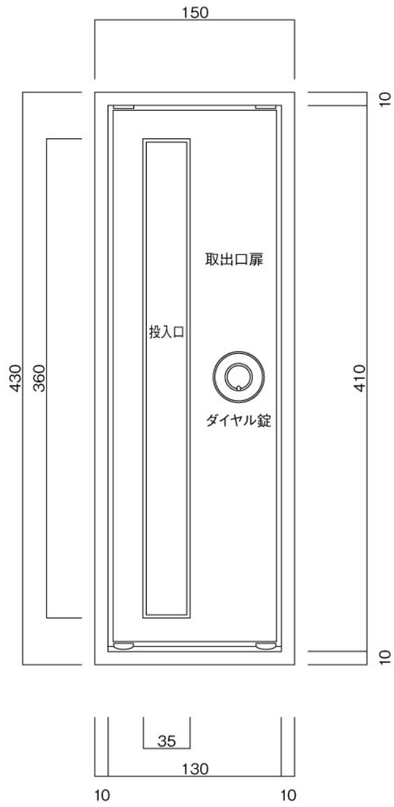
正面図
