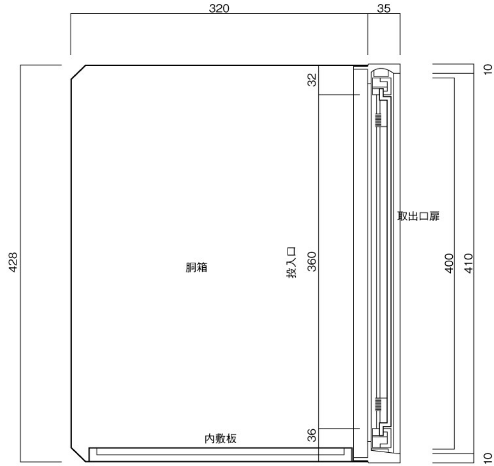
縦断面図
